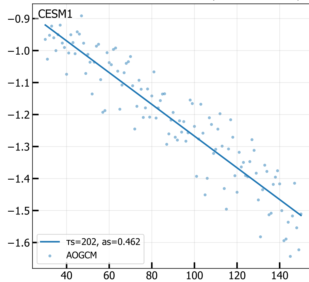
4xCO 2 log(T eq -T) - log(T eq ) vs. Time (slow mode, iter 3)
