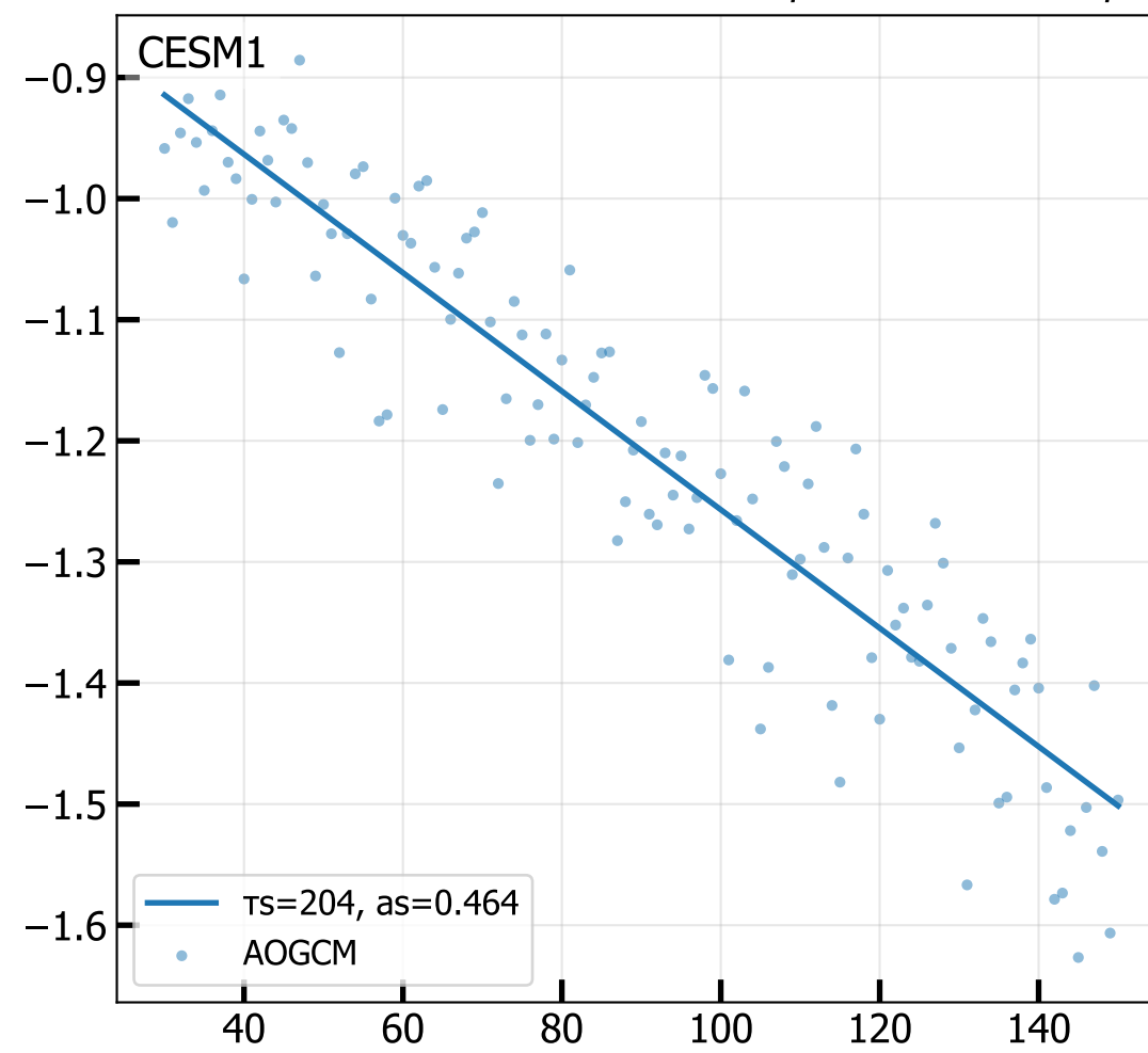
4xCO 2 log(T eq -T) - log(T eq ) vs. Time (slow mode, iter 4)
