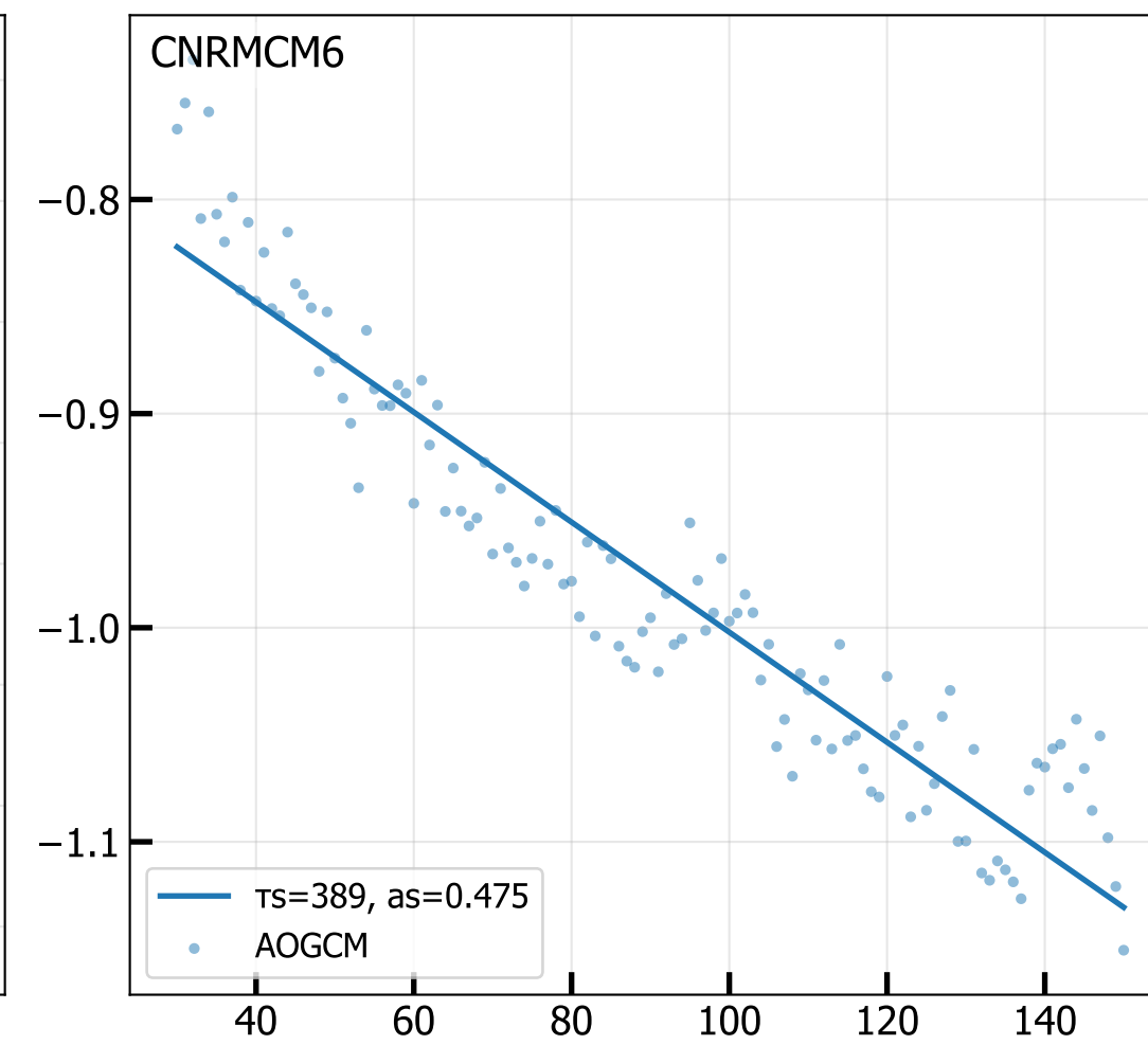
4xCO 2 log(T eq -T) - log(T eq ) vs. Time (slow mode, iter 7)
