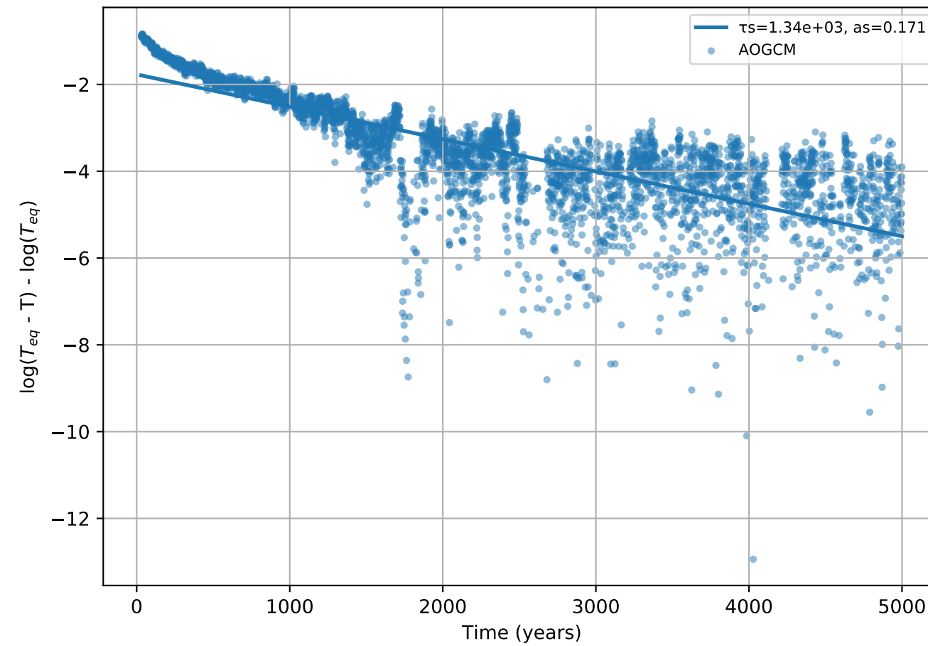
GISSE2R: slow mode, iter 9
