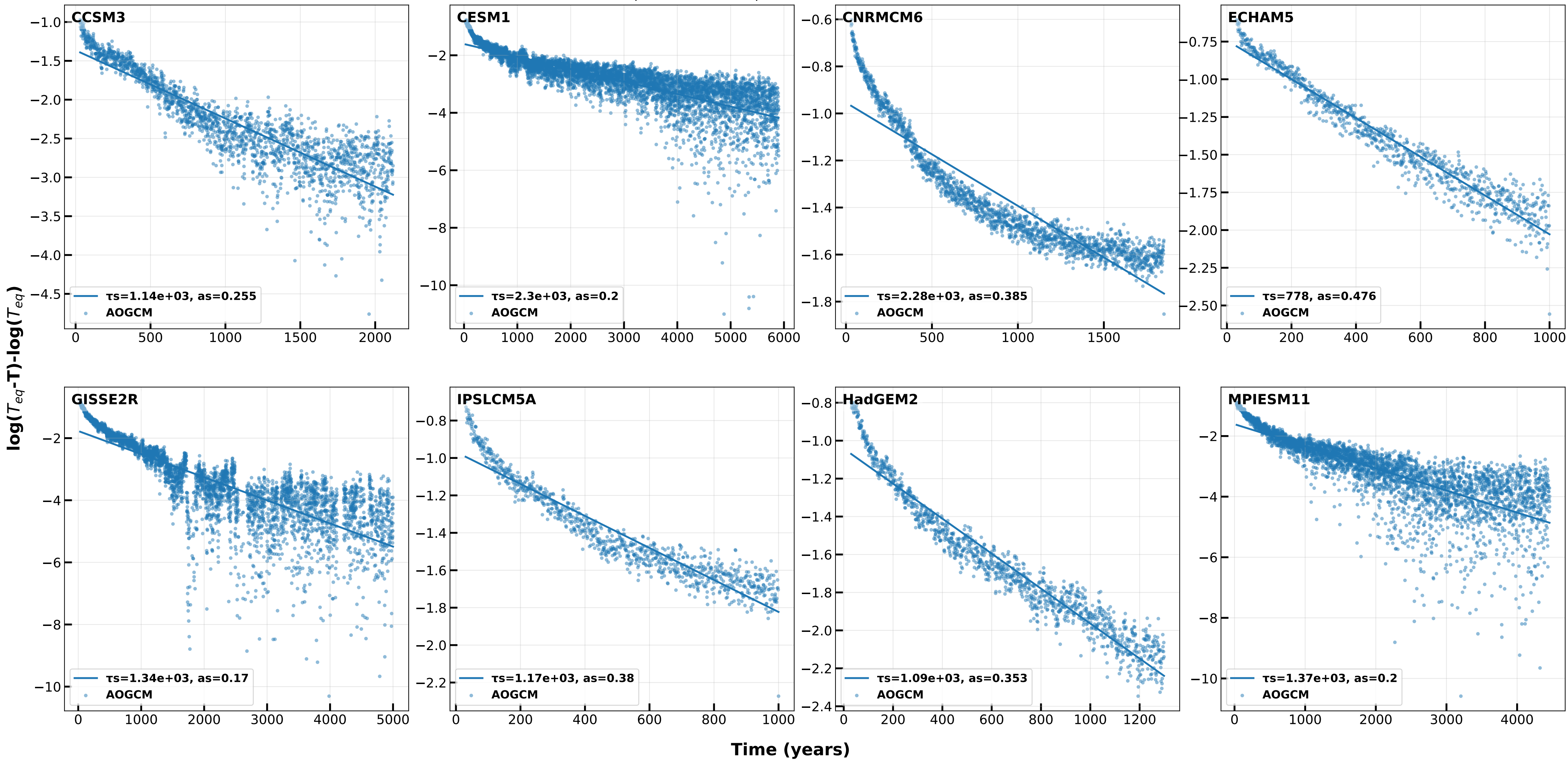
4xCO 2 log(T eq -T) - log(T eq ) vs. Time (slow mode, iter 10)
