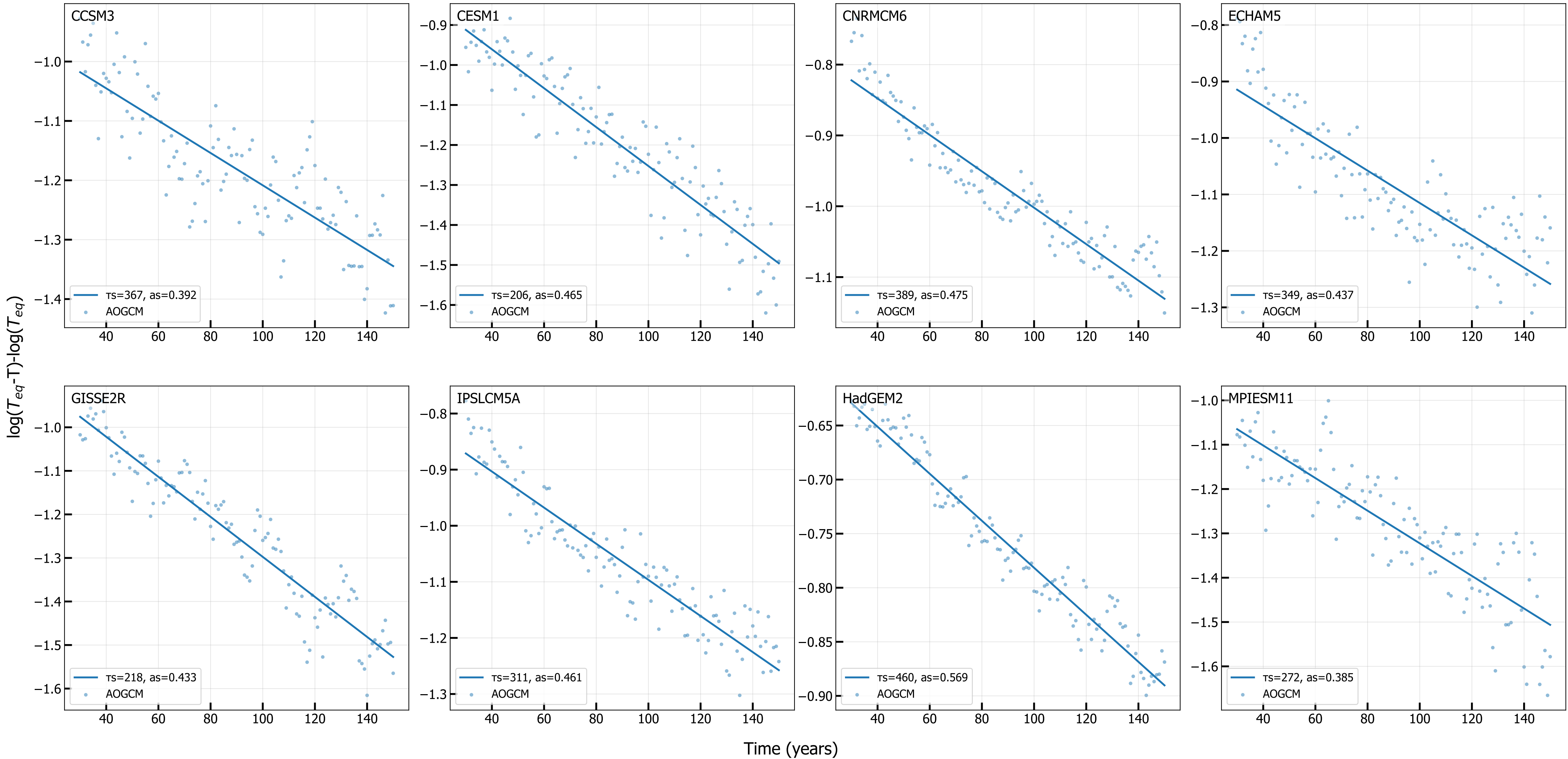
4xCO 2 log(T eq -T) - log(T eq ) vs. Time (slow mode, iter 6)
