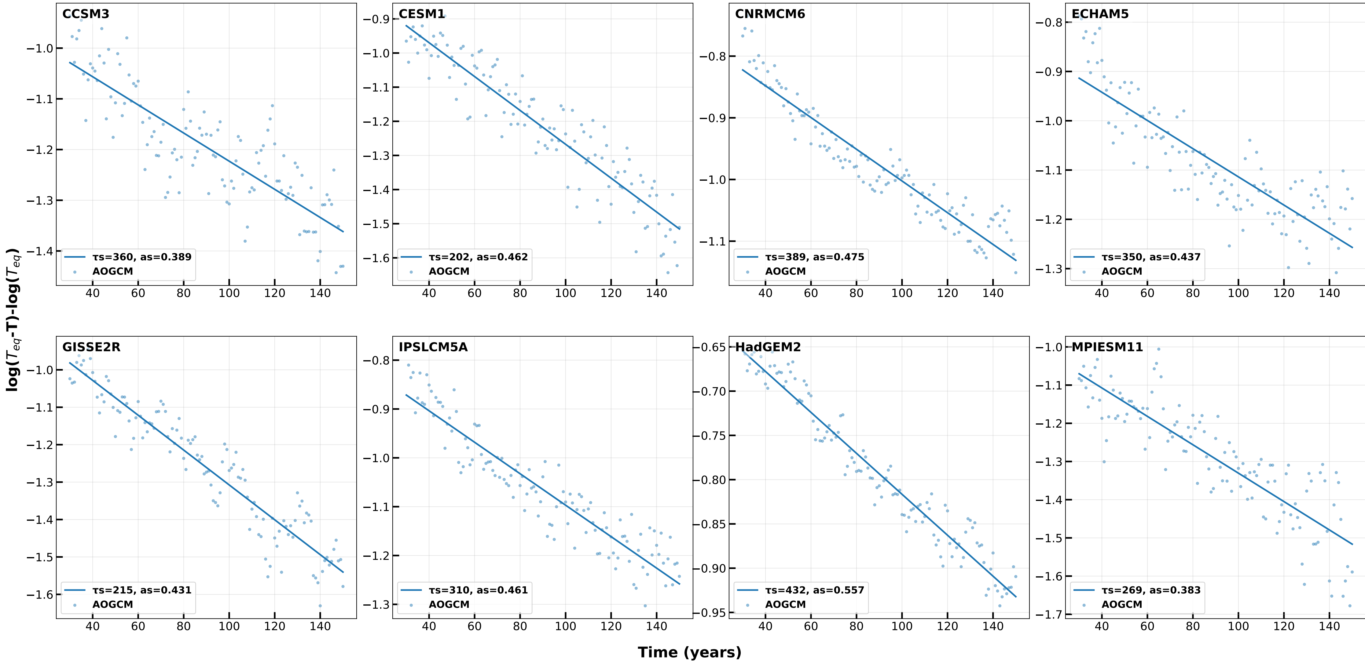
4xCO 2 log(T eq -T) - log(T eq ) vs. Time (slow mode, iter 3)
