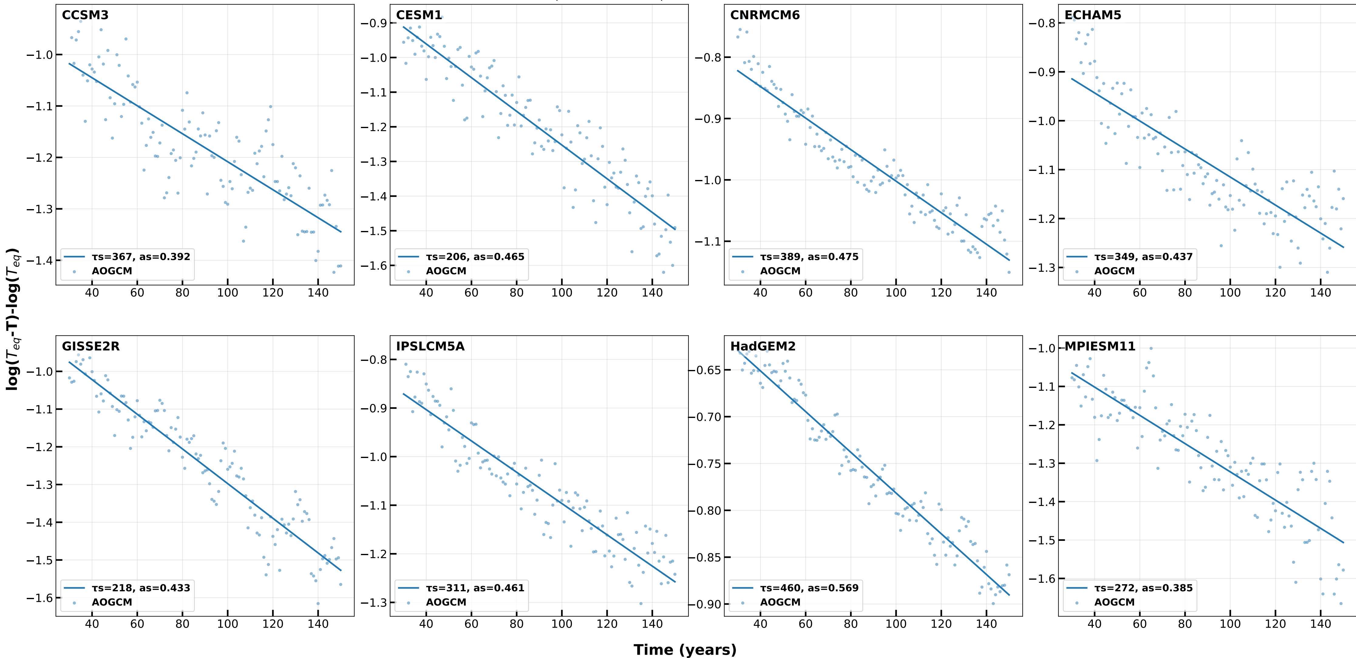
4xCO 2 log(T eq -T) - log(T eq ) vs. Time (slow mode, iter 6)
