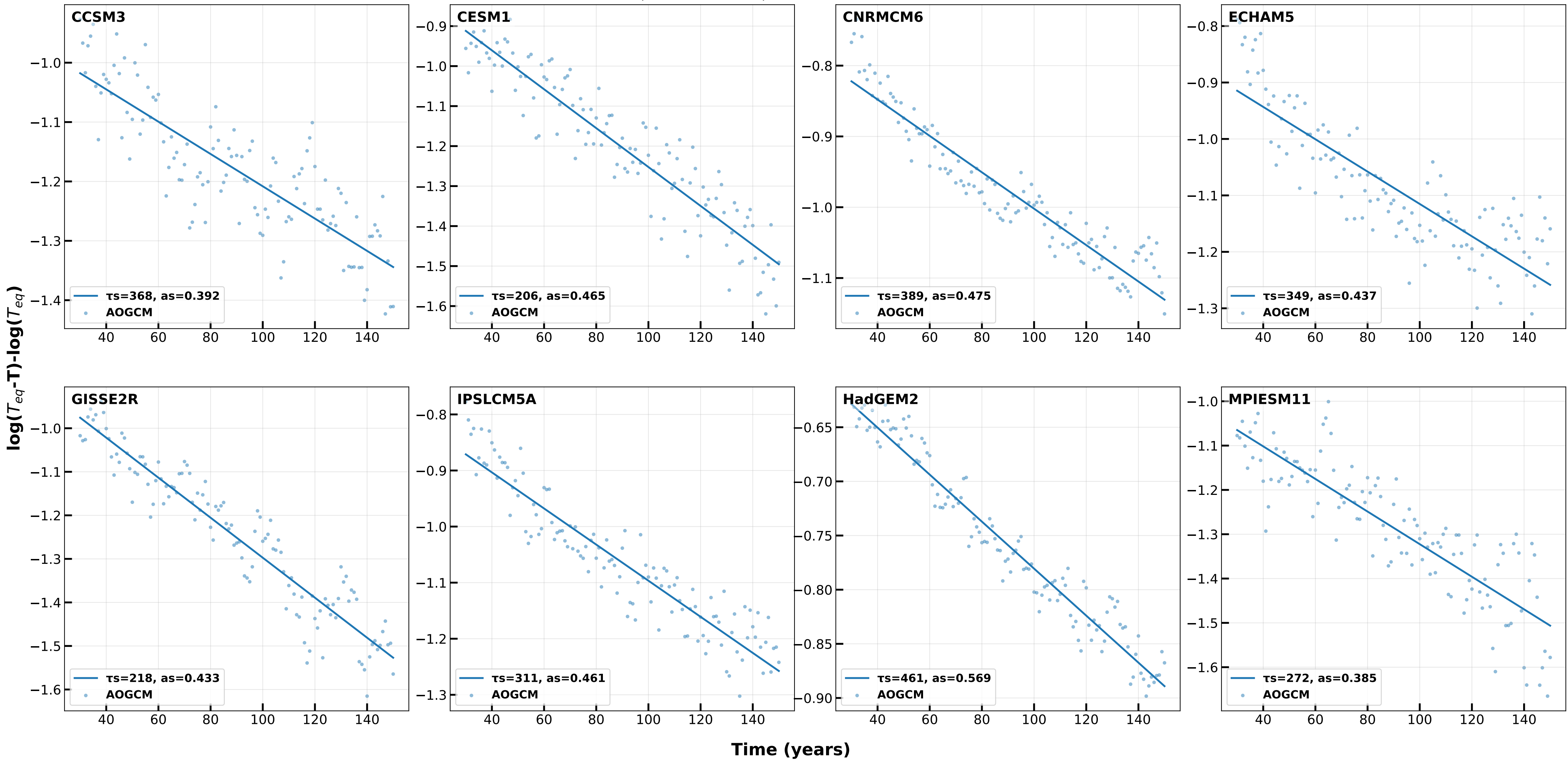
4xCO 2 log(T eq -T) - log(T eq ) vs. Time (slow mode, iter 7)
