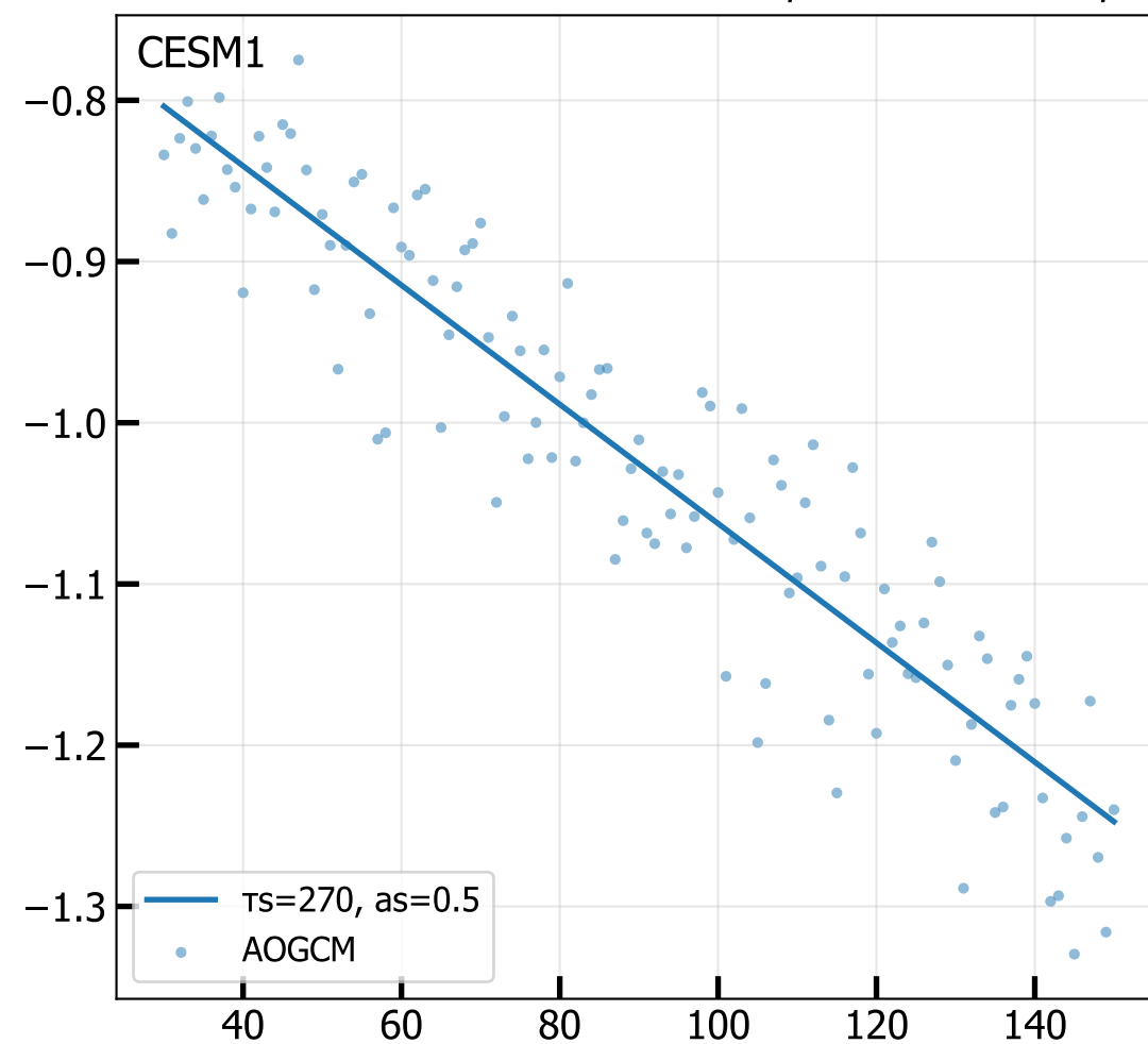
4xCO 2 log(T eq -T) - log(T eq ) vs. Time (slow mode, iter 9)
