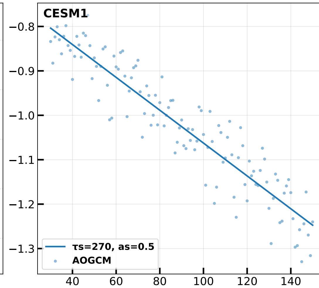
4xCO 2 log(T eq -T) - log(T eq ) vs. Time (slow mode, iter 8)
