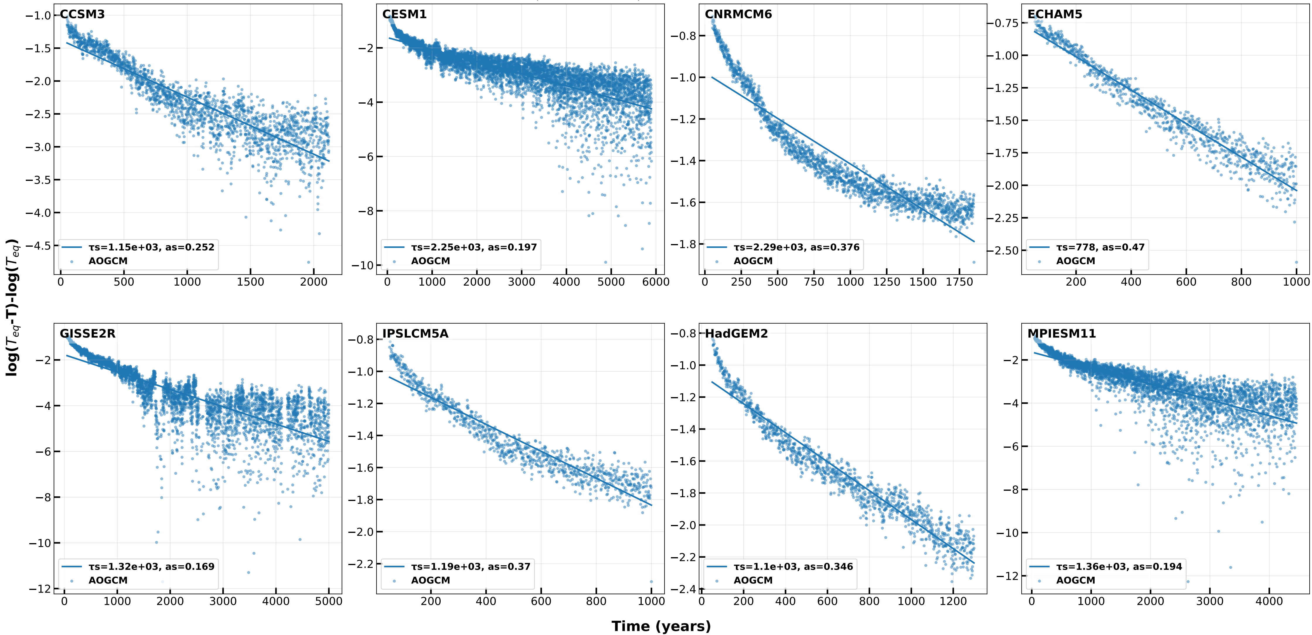
4xCO 2 log(T eq -T) - log(T eq ) vs. Time (slow mode, iter 2)
