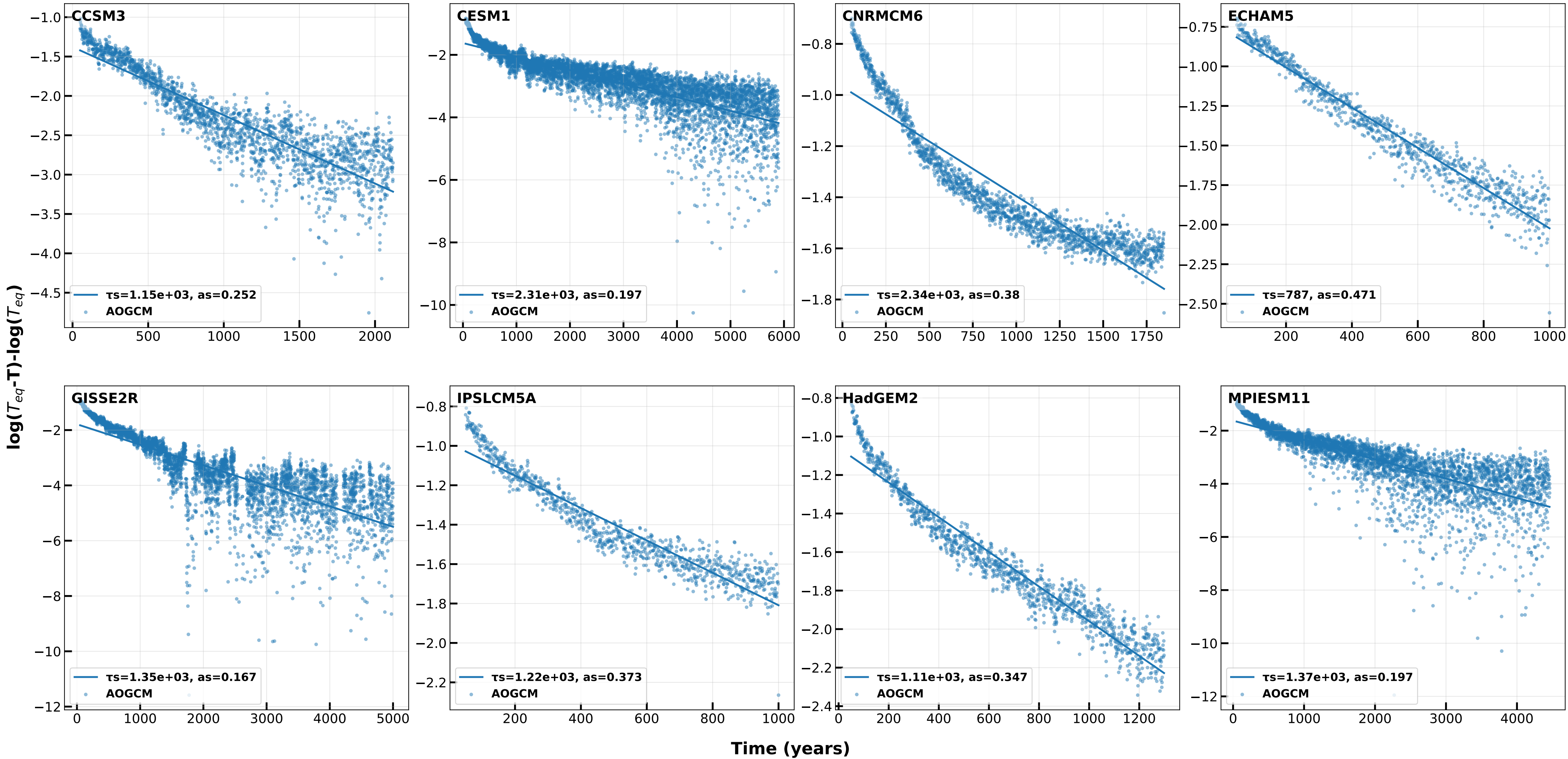
4xCO 2 log(T eq -T) - log(T eq ) vs. Time (slow mode, iter 3)
