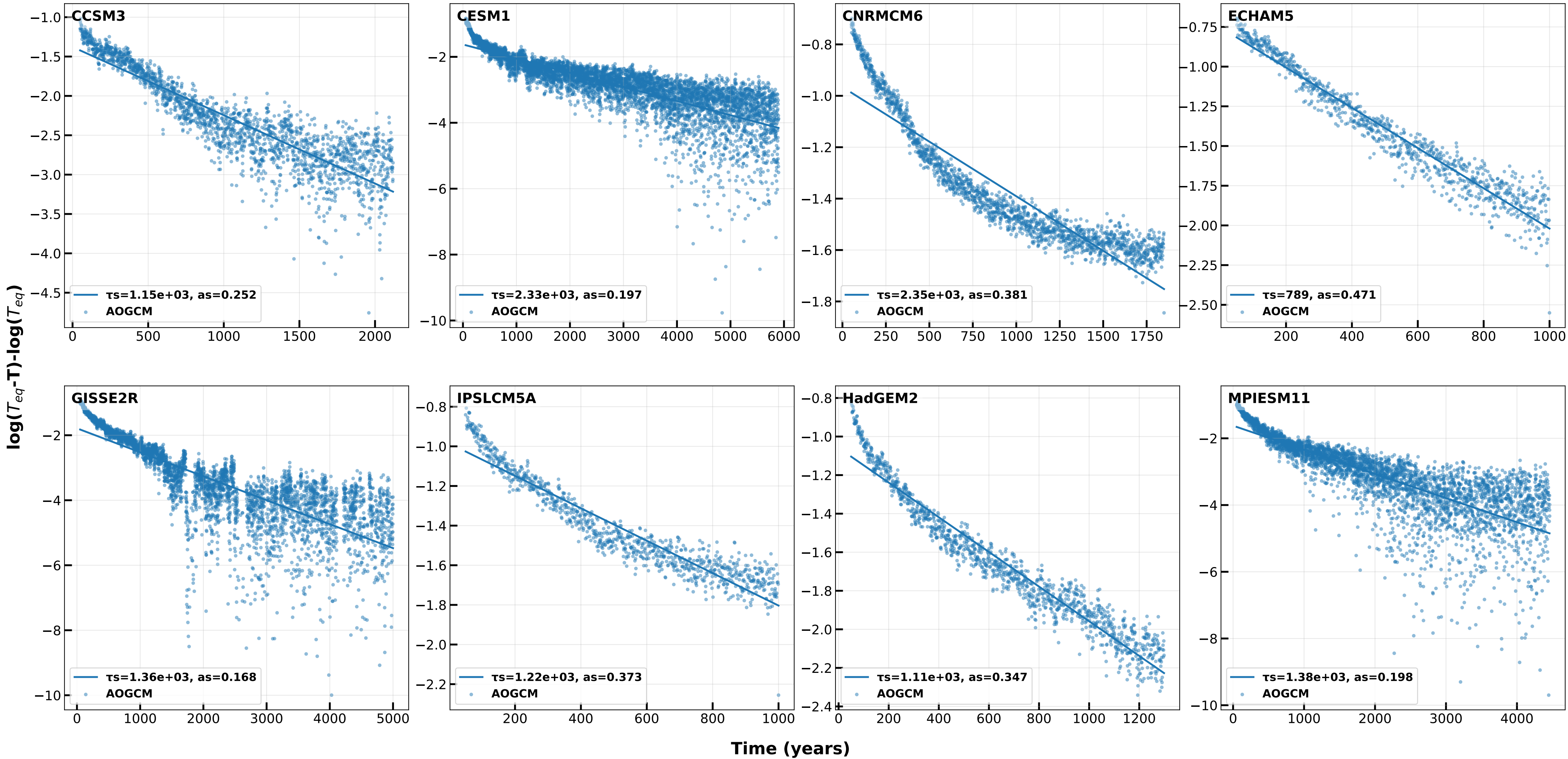
4xCO 2 log(T eq -T) - log(T eq ) vs. Time (slow mode, iter 4)
