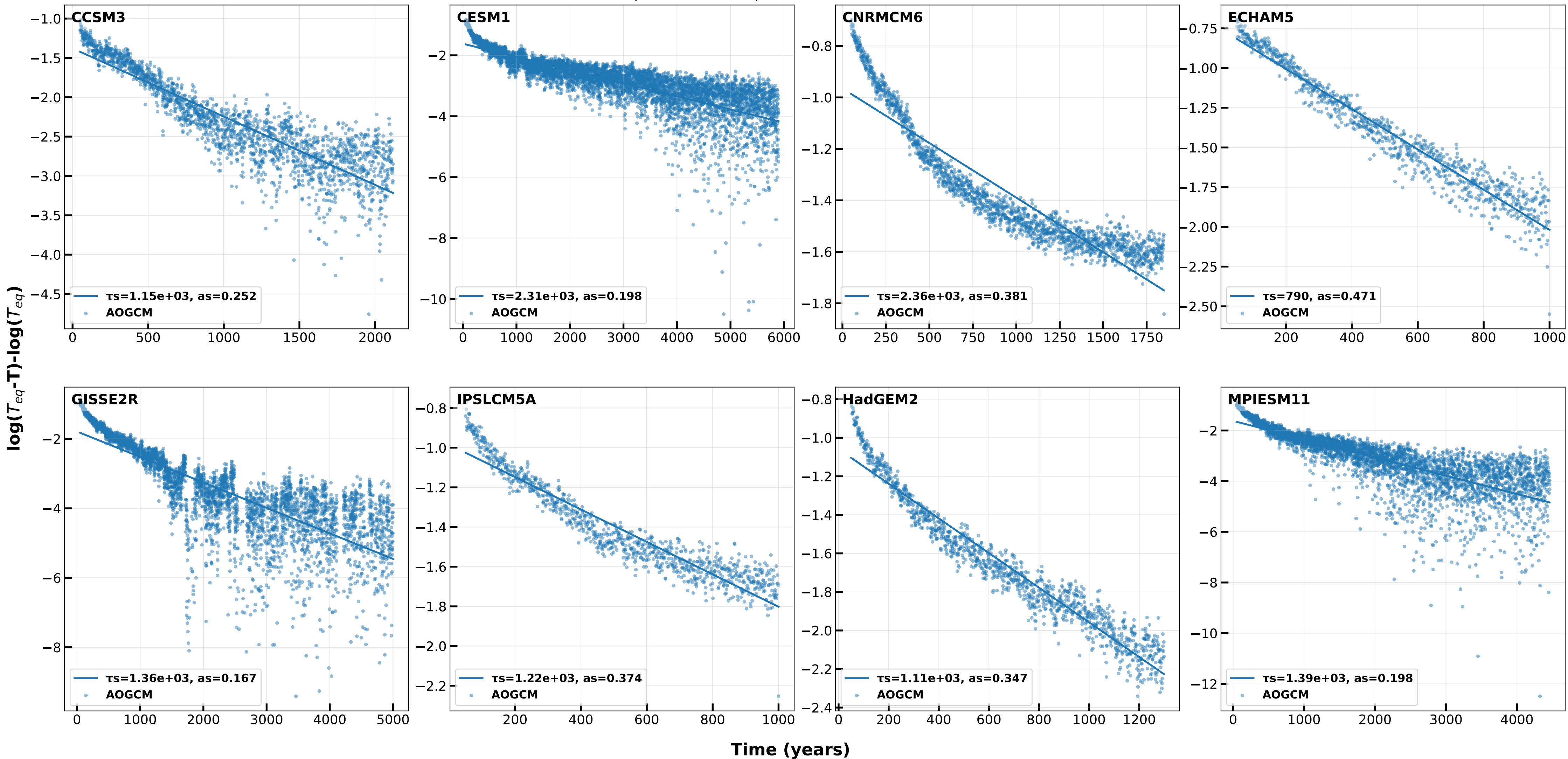
4xCO 2 log(T eq -T) - log(T eq ) vs. Time (slow mode, iter 10)
