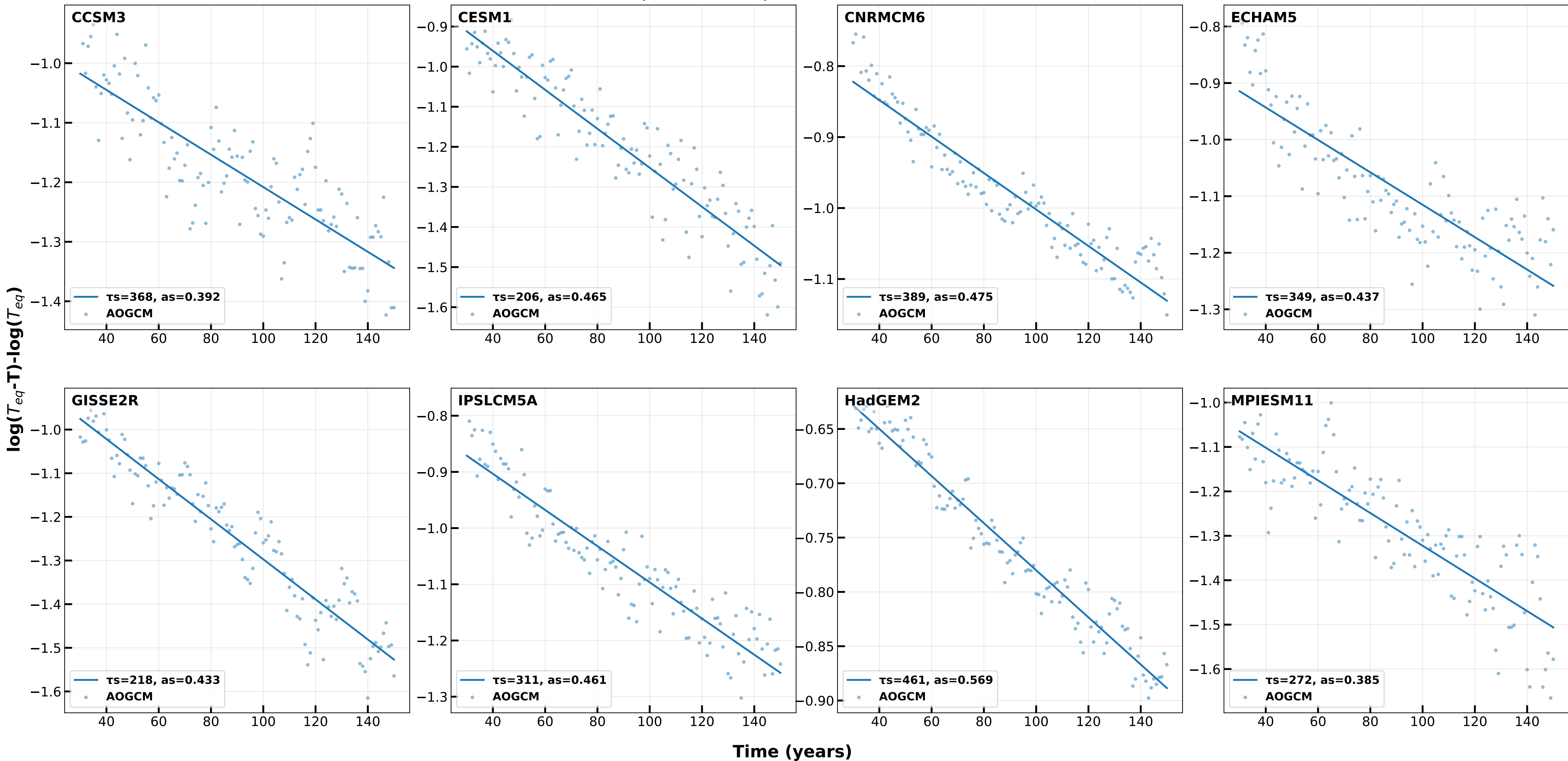
4xCO 2 log(T eq -T) - log(T eq ) vs. Time (slow mode, iter 9)
