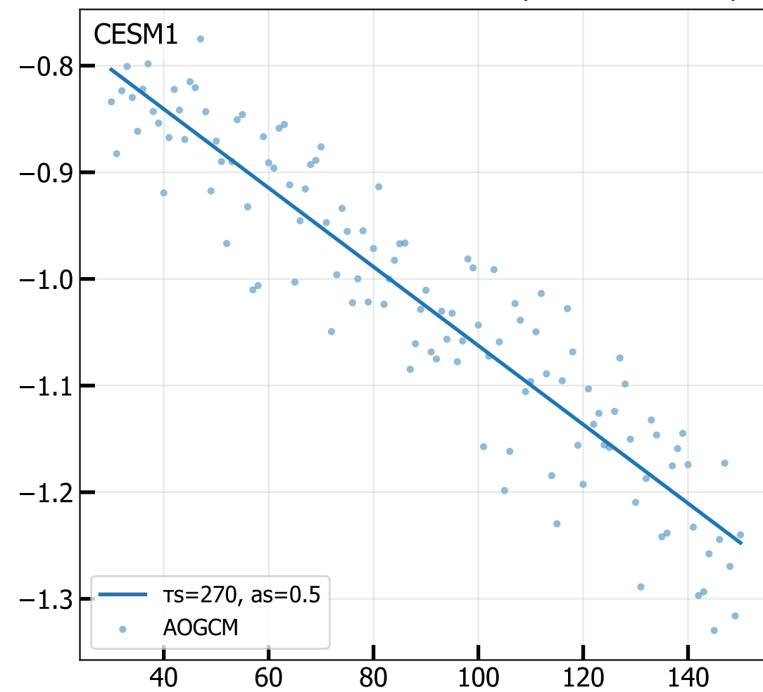
4xCO 2 log(T eq -T) - log(T eq ) vs. Time (slow mode, iter 5)
