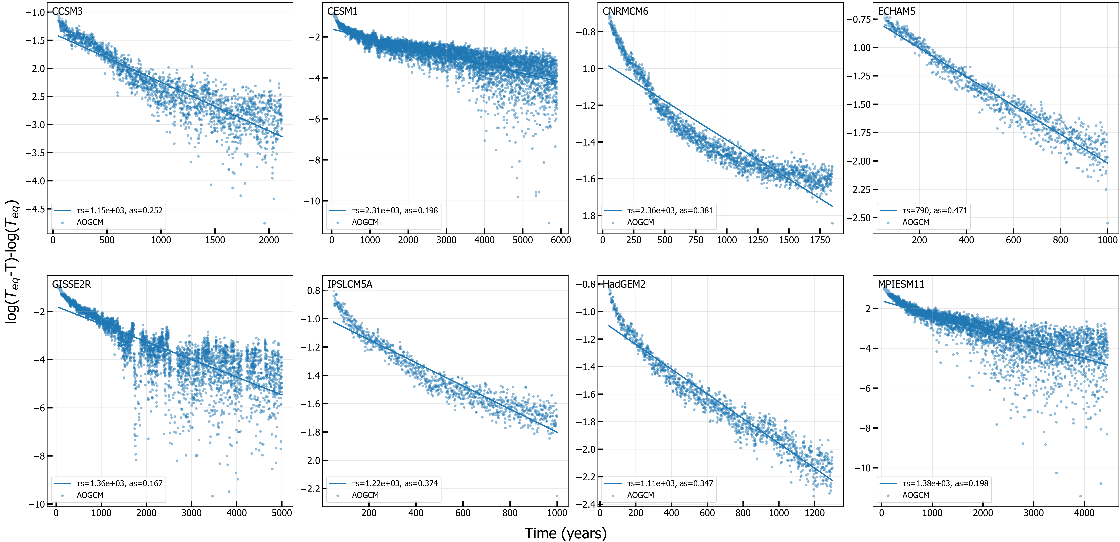
4xCO 2 log(T eq -T) - log(T eq ) vs. Time (slow mode, iter 7)
