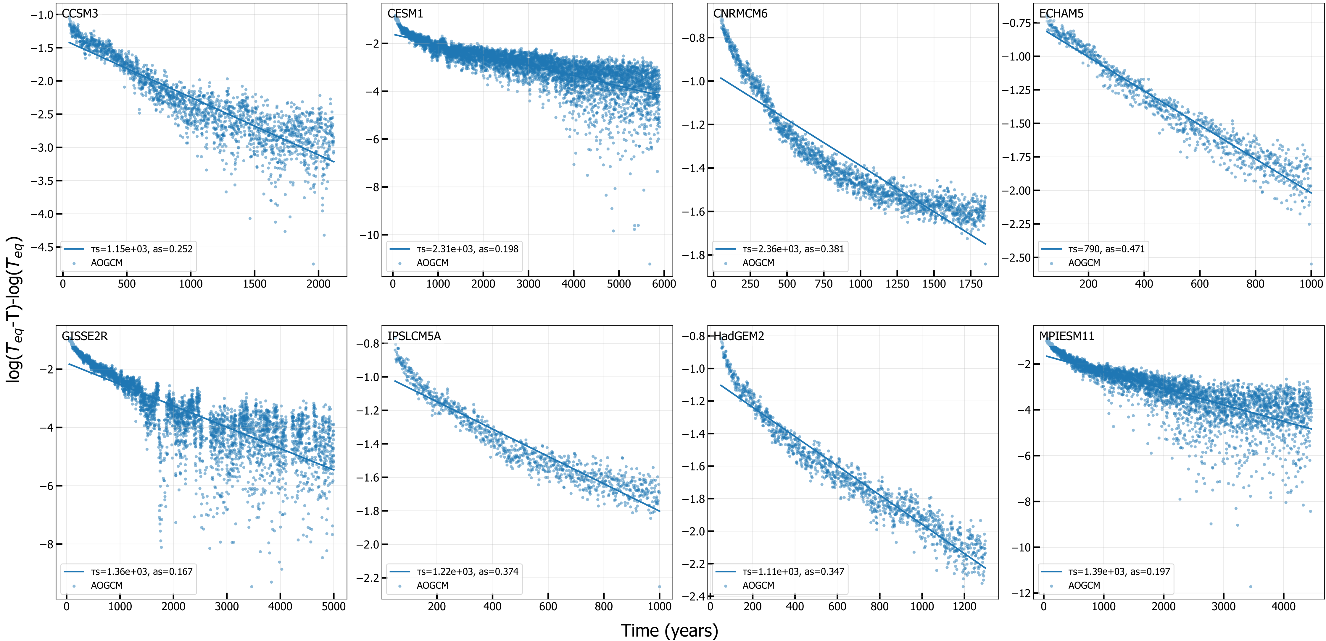
4xCO 2 log(T eq -T) - log(T eq ) vs. Time (slow mode, iter 9)
