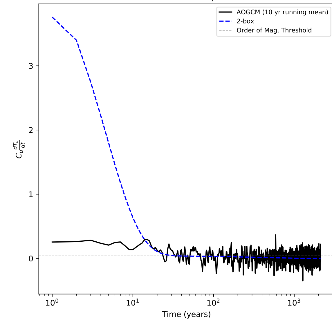
GISSE2R 4xCO2: Assumption 2 Test
