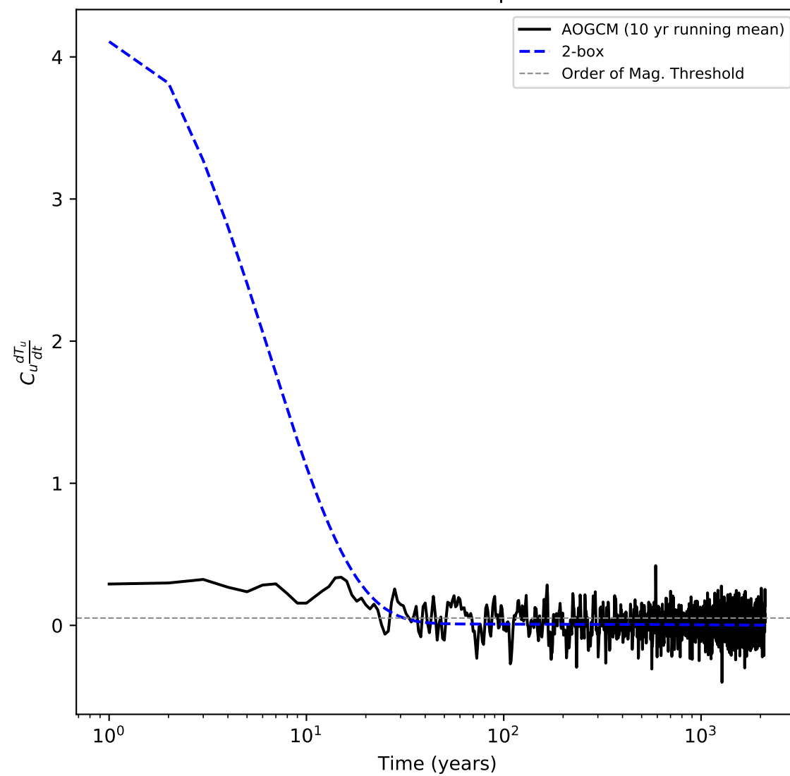
GISSE2R 4xCO2: Assumption 2 Test
