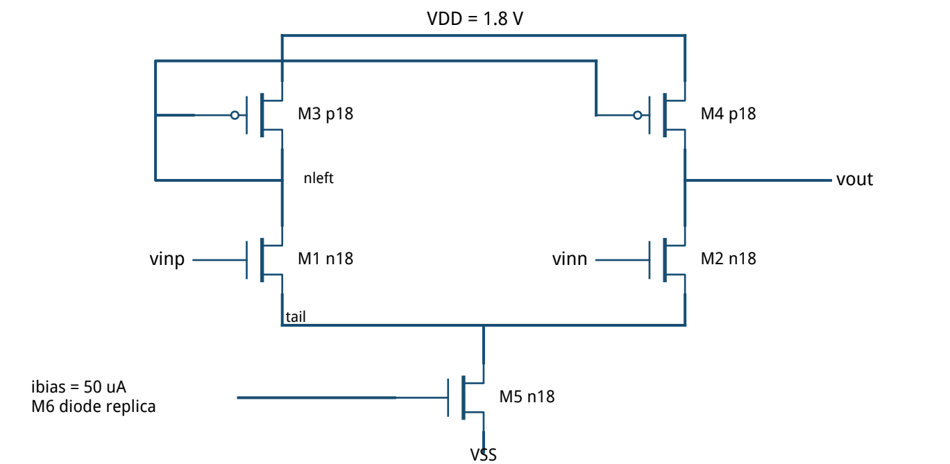
图示为信号核心。M6与M5共栅偏置；体端与完整端序见第4页网表。
