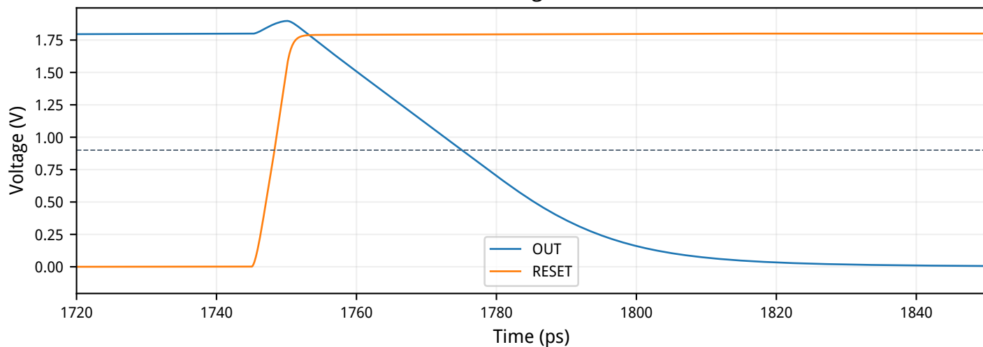
Reset edge detail
