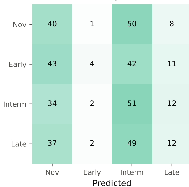
Dance — Qwen3-VL
