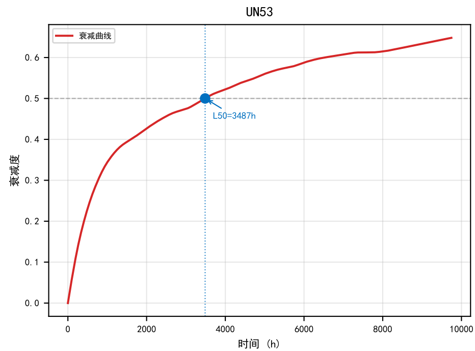
105℃ LED衰减度扩充曲线 & L50标注（外推按末段斜率）
