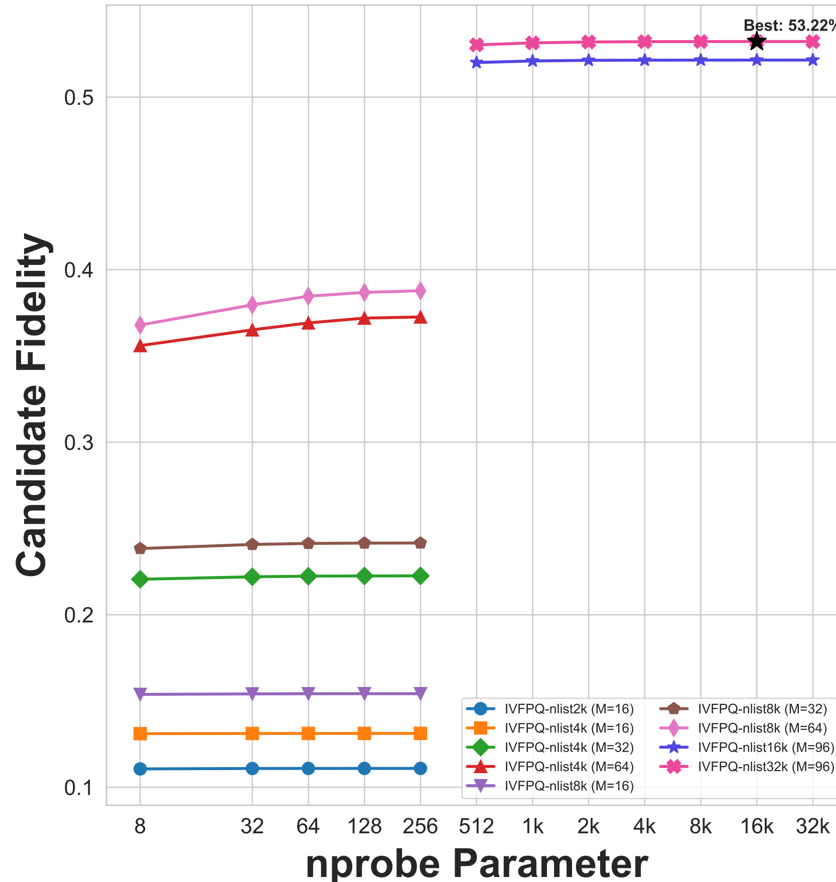
(b) IVFPQ
