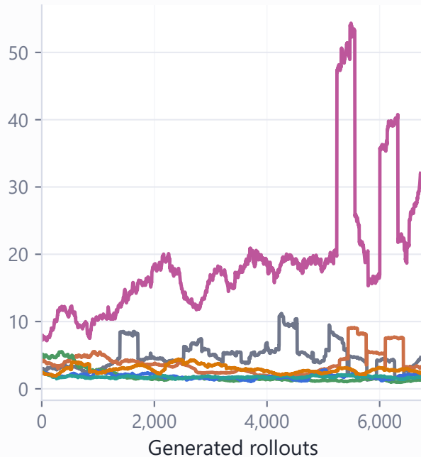
Gradient norm
