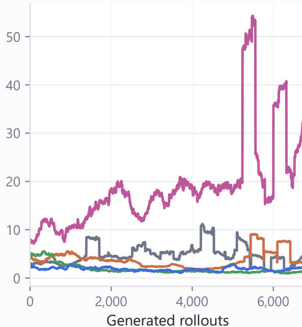
Gradient norm
