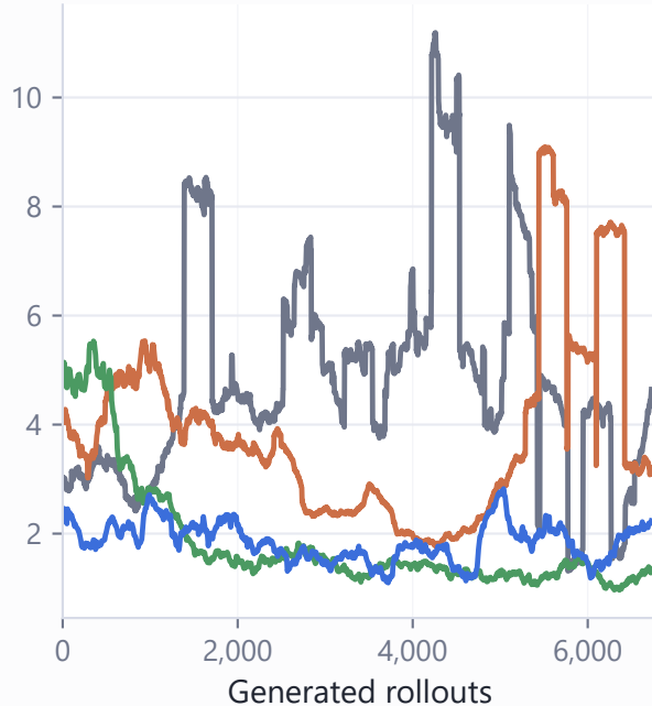
Gradient norm
