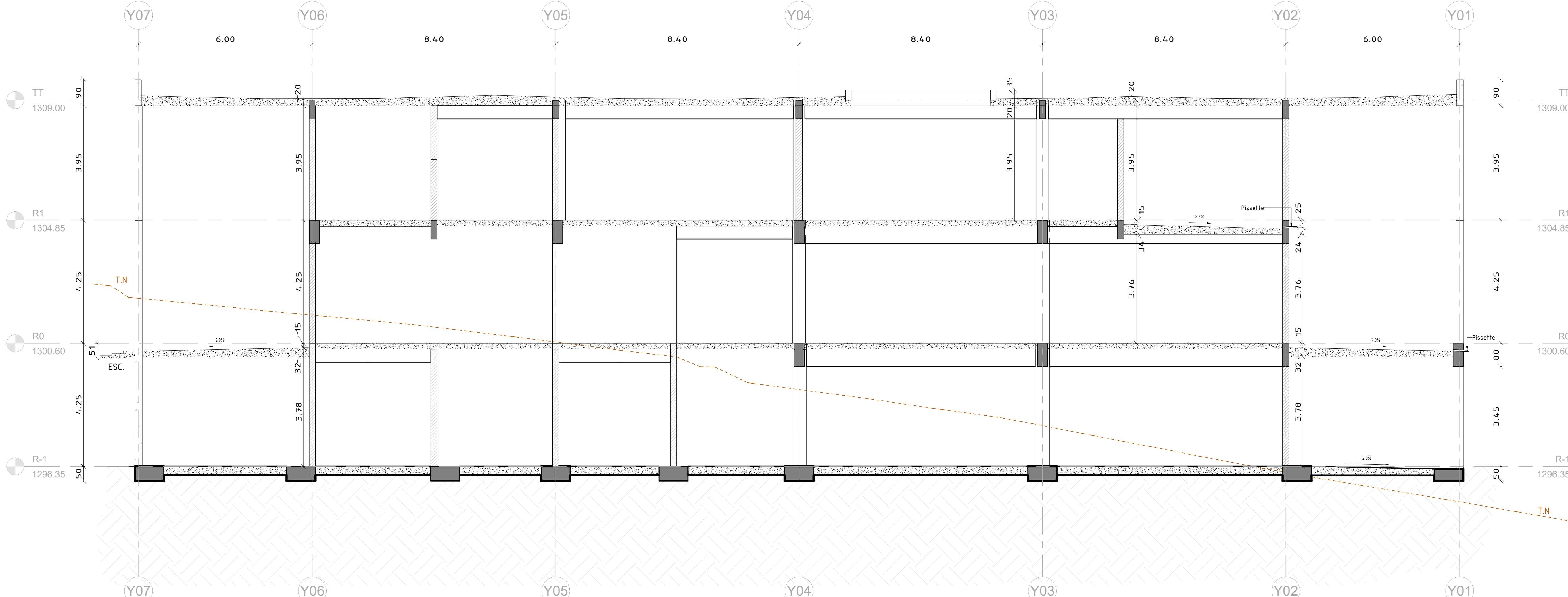
COUPE BB'
