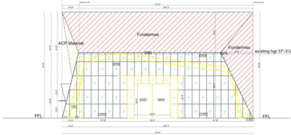
ELEVATION A
