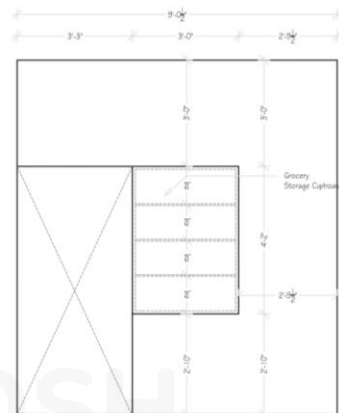
D-side
