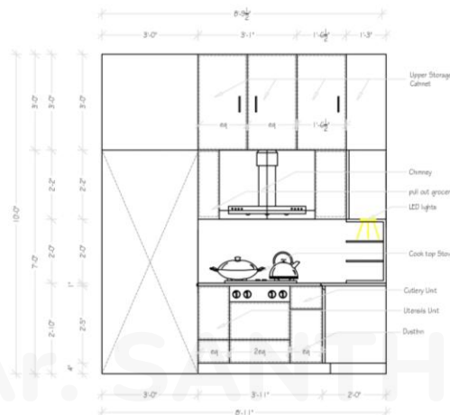
C-side
