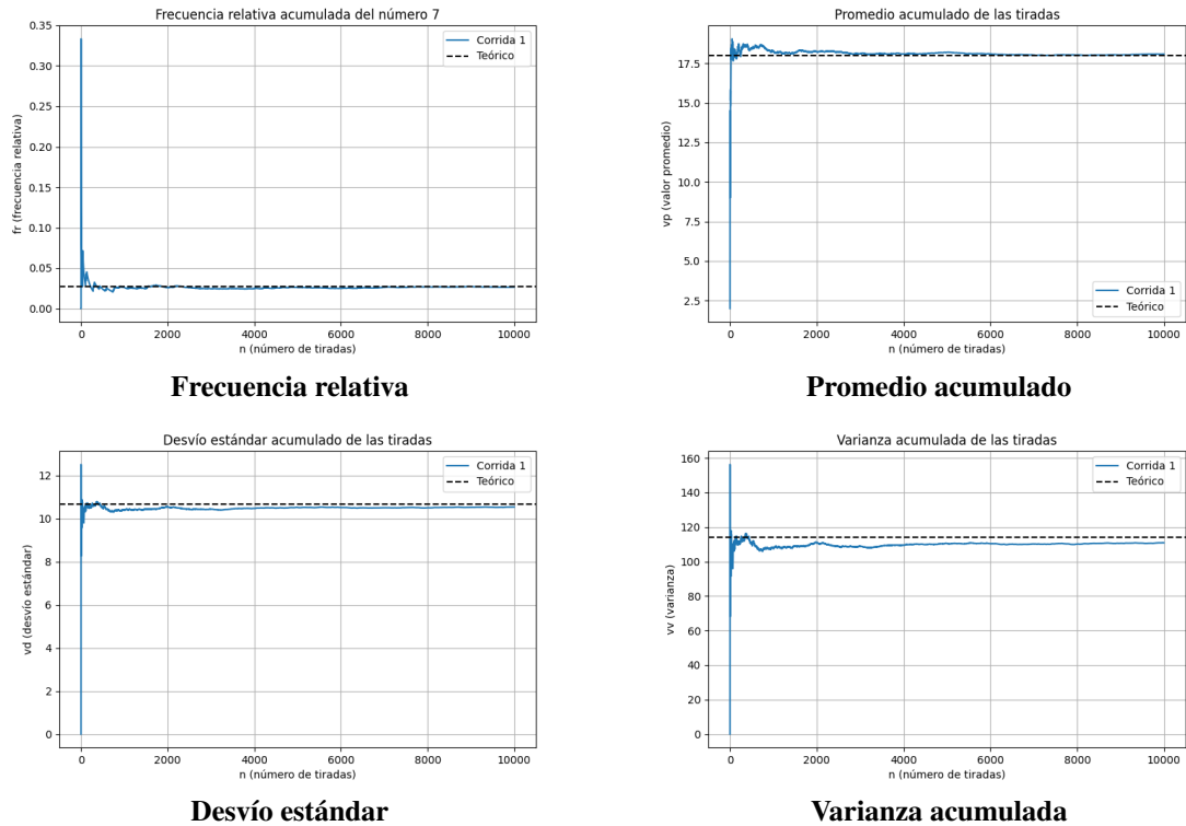
Figure 4: Métricas estadísticas obtenidas con 1 corrida.
