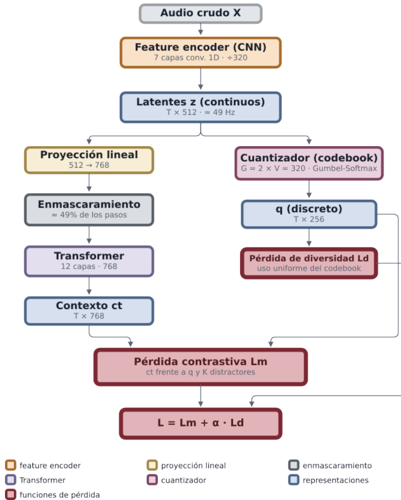
Fig. 1. Flujo del Preentrenamiento de Wav2Vec 2.0
