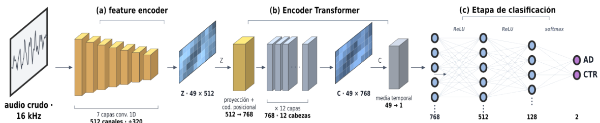
Fig 2: Arquitectura de Wav2Vec 2.0 para clasificación: (a) feature encoder, (b) encoder Transformer y (c) Etapa de clasificación.
