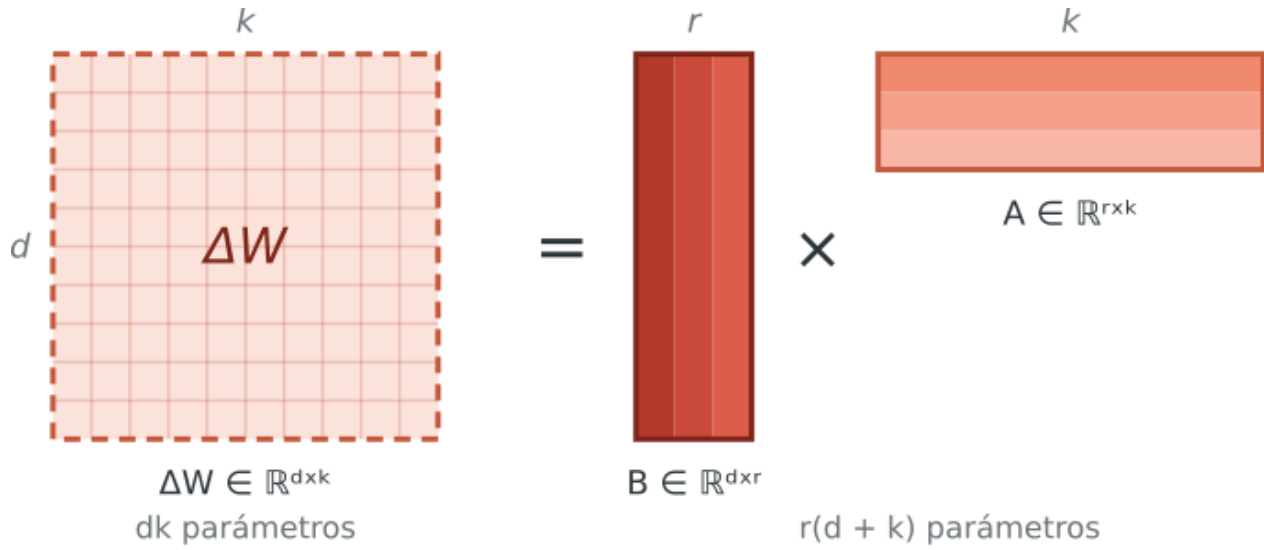
Fig. 5. Factorización de rango de la actualización de pesos \Delta W en las matrices de bajo rango B y A .
