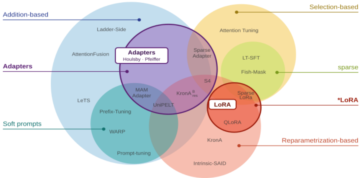
Fig. 3. Taxonomía de métodos PEFT, con los adapters y LoRA resaltados. Adaptada de Lialin et al. [16].
