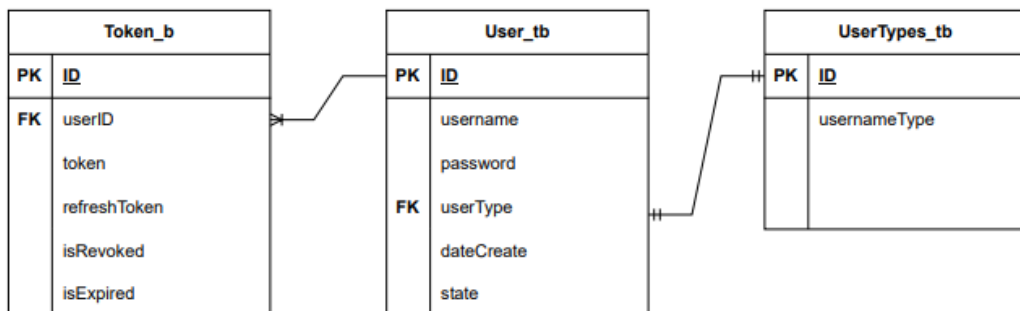
DIAGRAMA DE BASE DE DATOS: ClandeStock_BD
