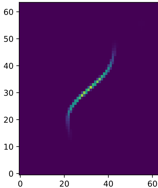
CVAE-GNO Pred
