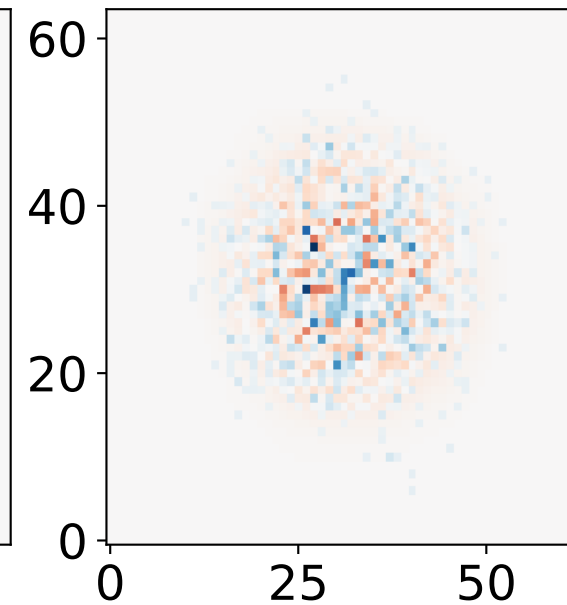
GNO Error
