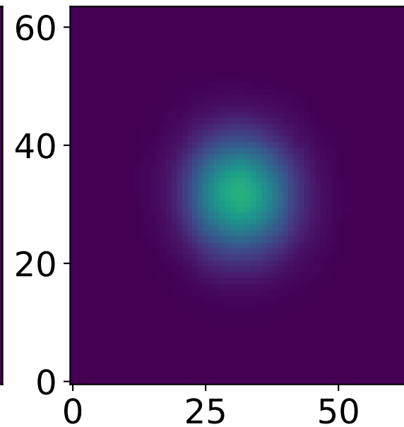
GNO Pred
