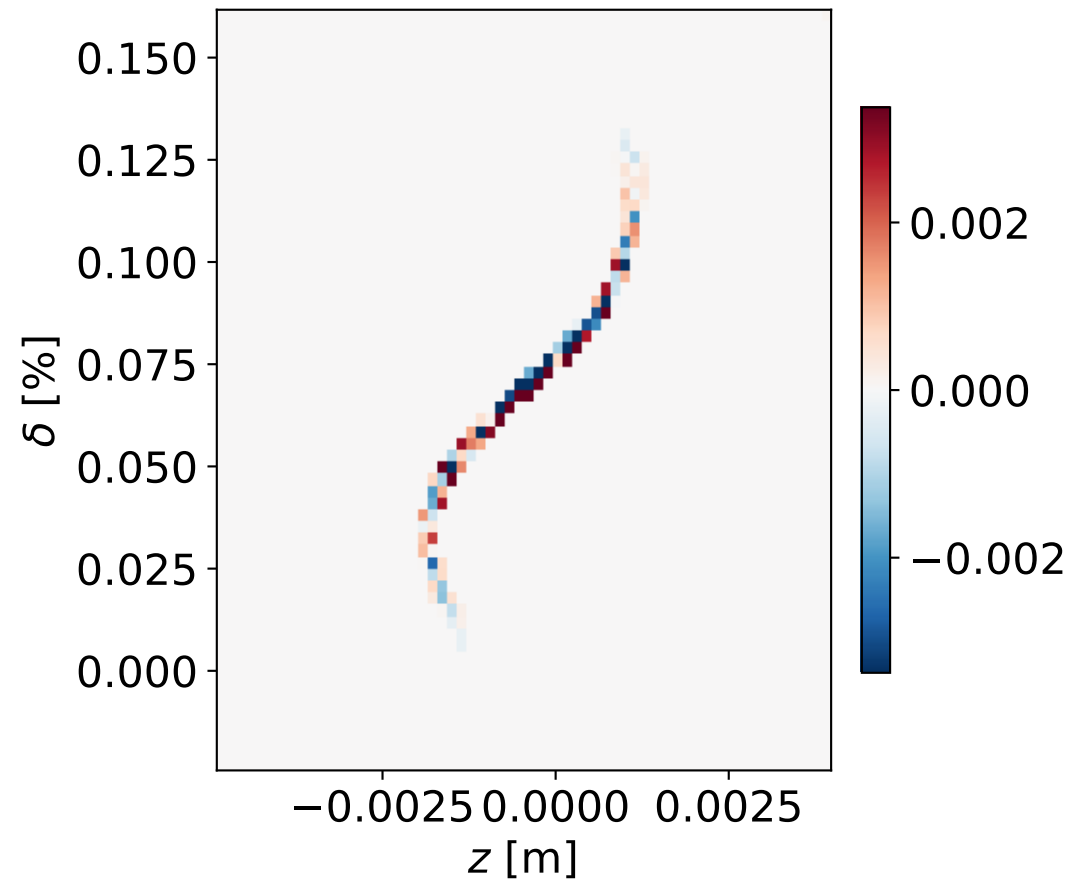
Pred - Truth
