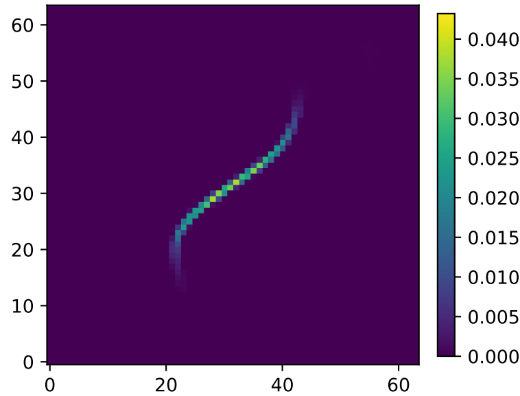
Pred
