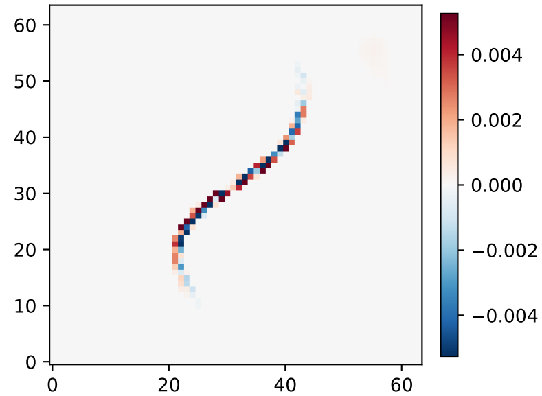
Pred - Truth
