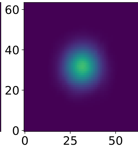
GNO Pred
