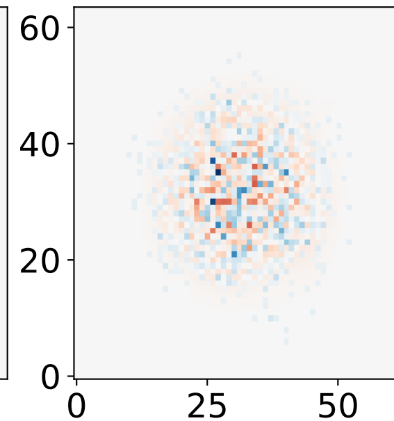
GNO Error
