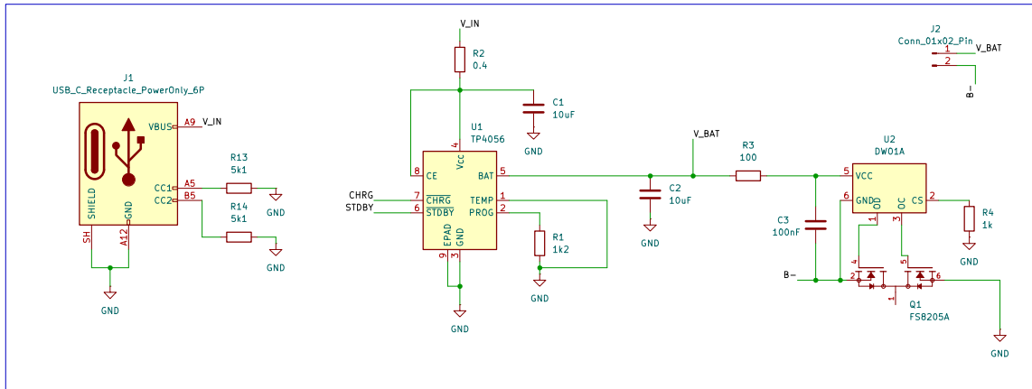
Circuito cargador de batería
