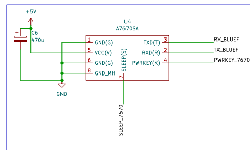
A7670SA comunicación GNSS+4G
