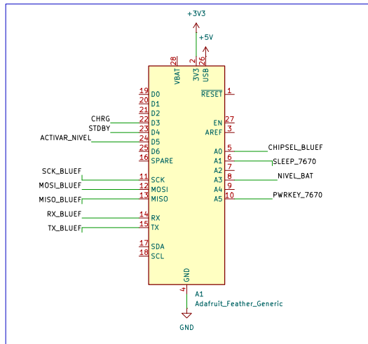
uC Bluefruit feather nrf52840 sense
