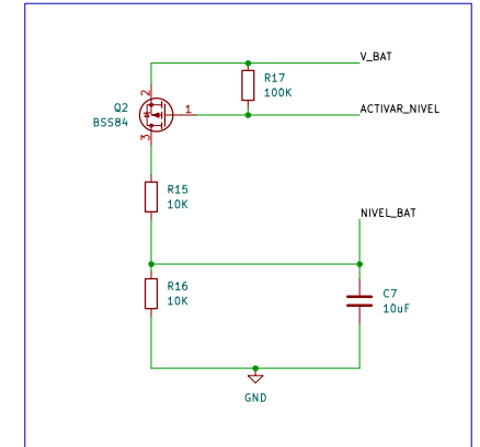
Circuito medidor nivel de Bat
