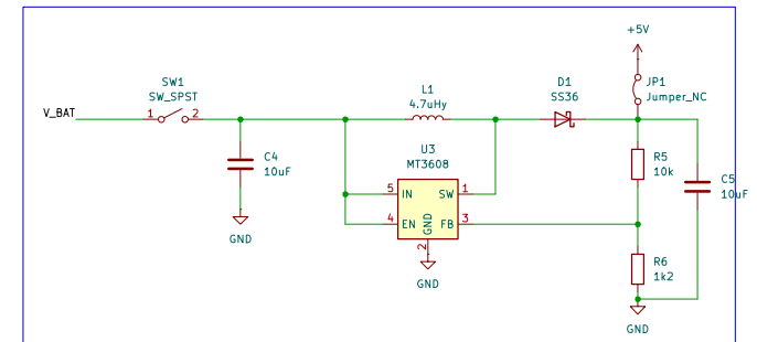
Circuito step-up // Vbat-->5V
