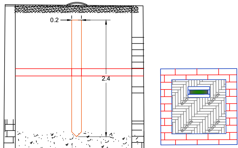
DETALLE CAMARA DE INSPECCION DE LA JABALINA
