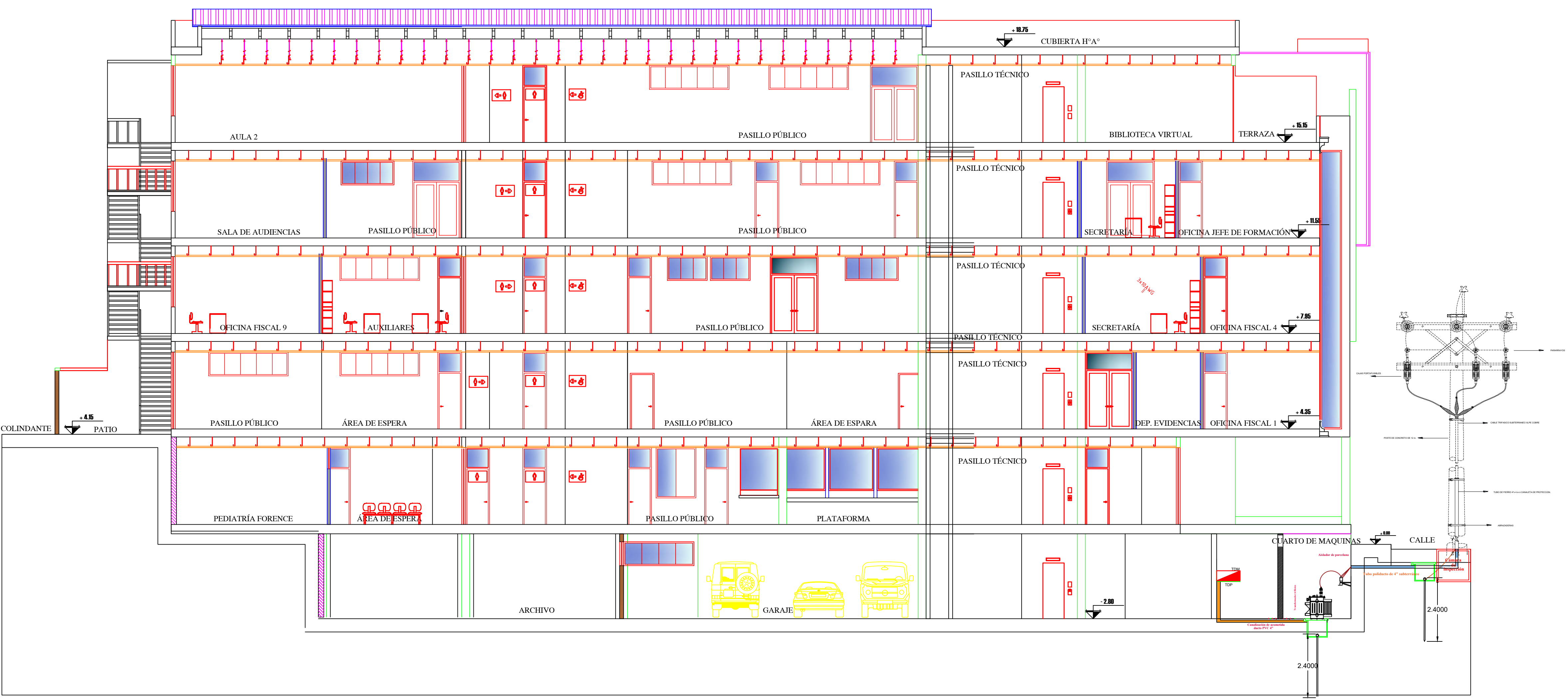
... CORTE A-A ... Esc. 1:50
