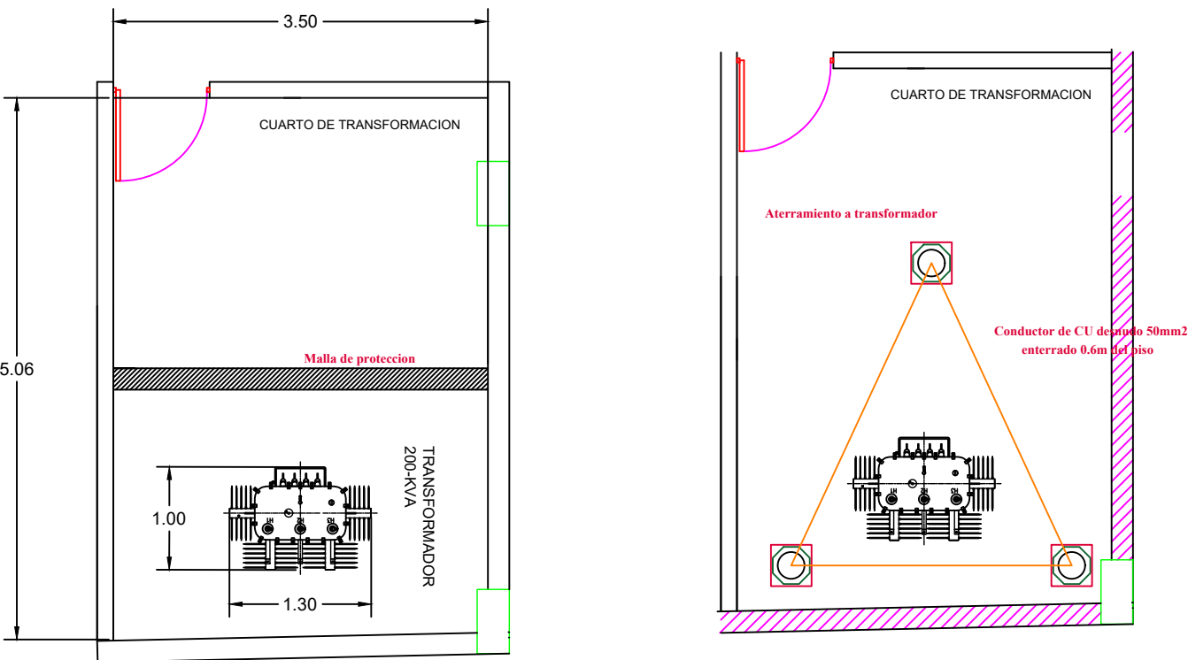
DETALLE CUARTO DE TRANSFORMACION
