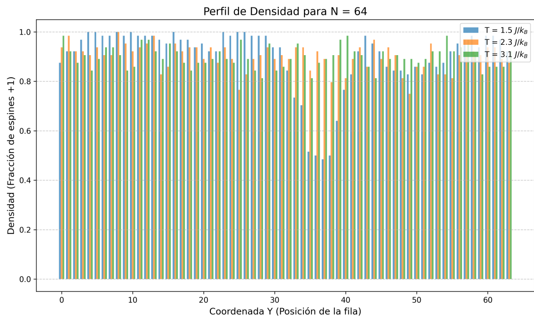
Figura 13: Densidad de partículas promedio en la dirección y para la red de 64x64 y a varias temperaturas.
