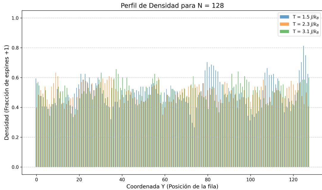
Figura 14: Densidad de partículas promedio en la dirección y para la red de 128 \times 128 y a varias temperaturas.
