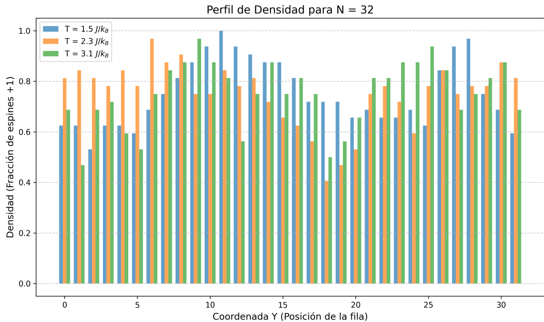
Figura 22: Densidad de partículas promedio en la dirección y para la red de 32 \times 32 y a varias temperaturas.
