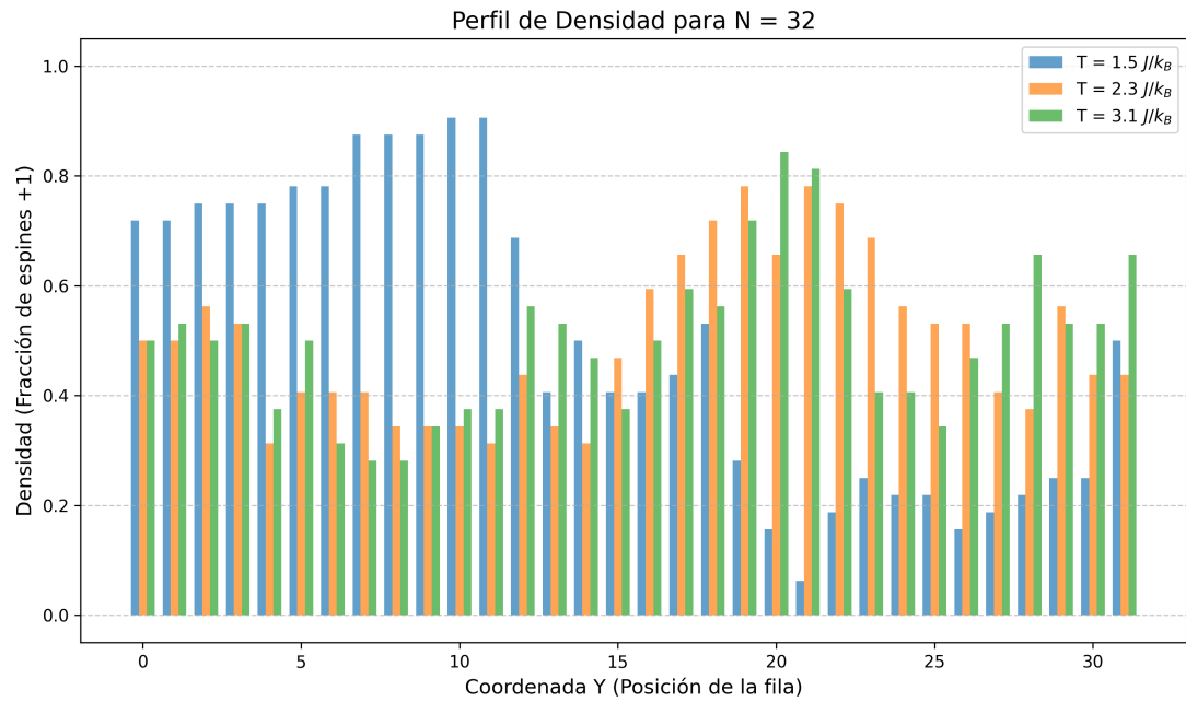
Figura 12: Densidad de partículas promedio en la dirección y para la red de 32x32 y a varias temperaturas.
