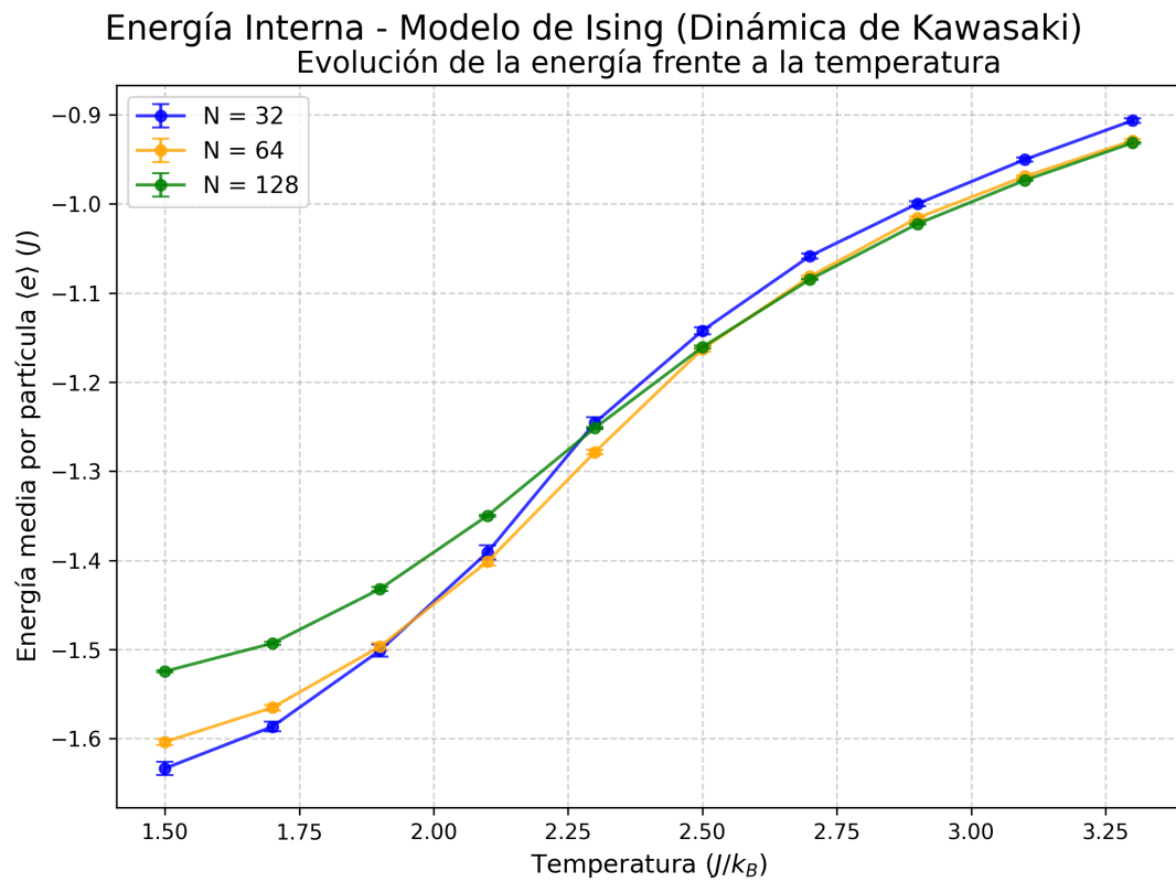
Figura 16: Energía media del sistema a distintas temperaturas y tamaños de red.
