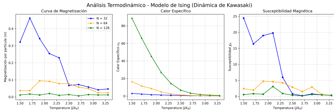
Figura 10: Curvas de magnetización, calor específico y susceptibilidad magnética frente a la temperatura para magnetización inicial nula.
