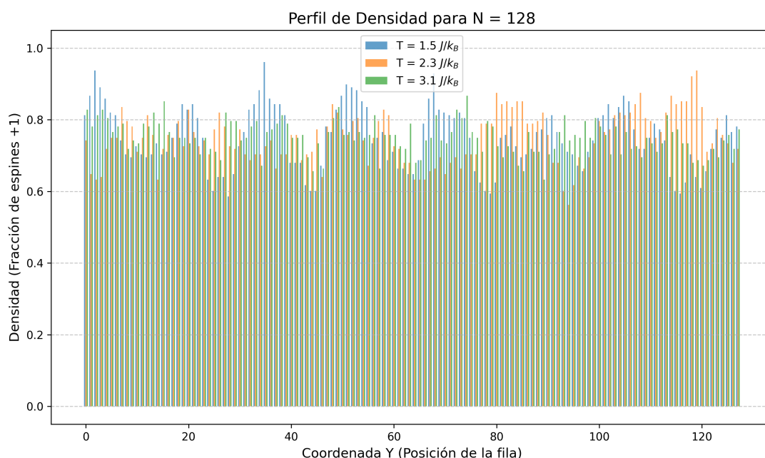
Figura 19: Densidad de partículas promedio en la dirección y para la red de 128x128 y a varias temperaturas.
