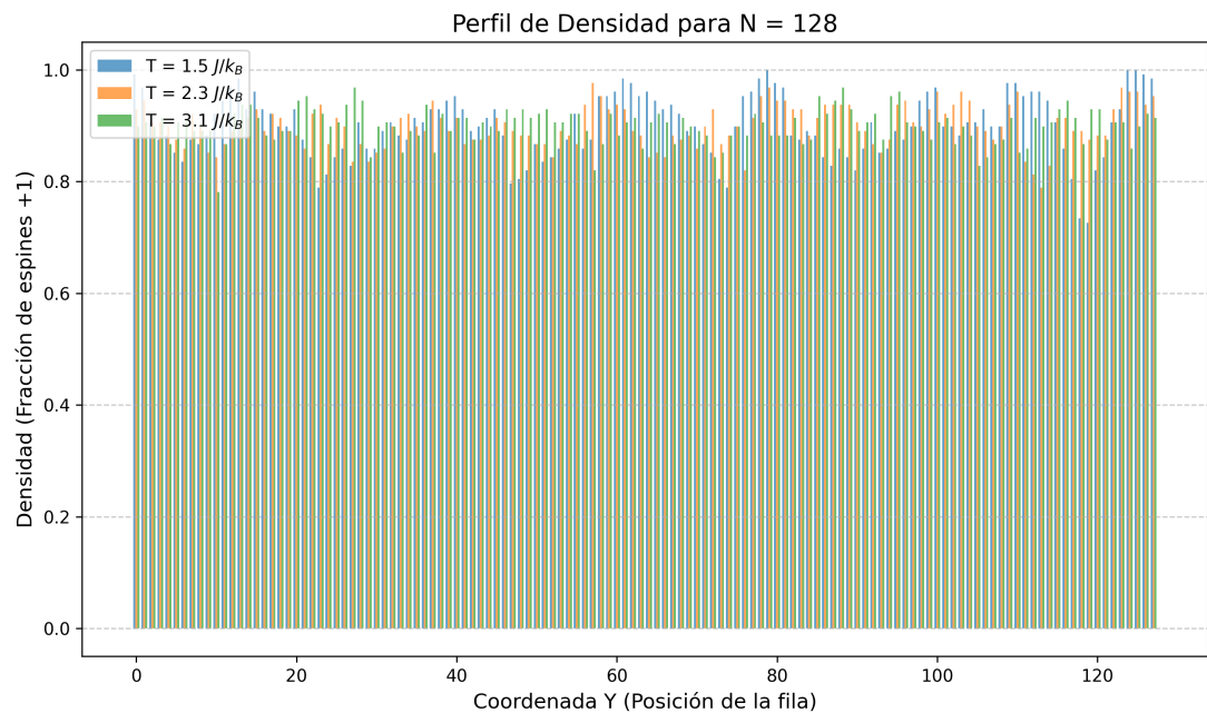
Figura 24: Densidad de partículas promedio en la dirección y para la red de 128x128 y a varias temperaturas.
