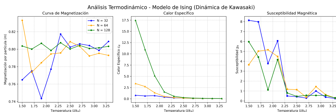
Figura 20: Curvas de magnetización, calor específico y susceptibilidad magnética frente a la temperatura para magnetización inicial de 0.8.
