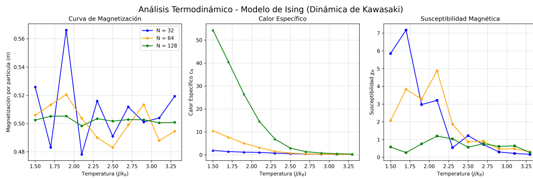
Figura 15: Curvas de magnetización, calor específico y susceptibilidad magnética frente a la temperatura para magnetización inicial de 0.5.
