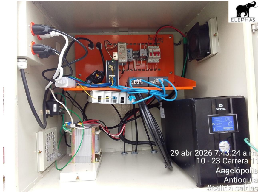
Foto Transformador Reductor
