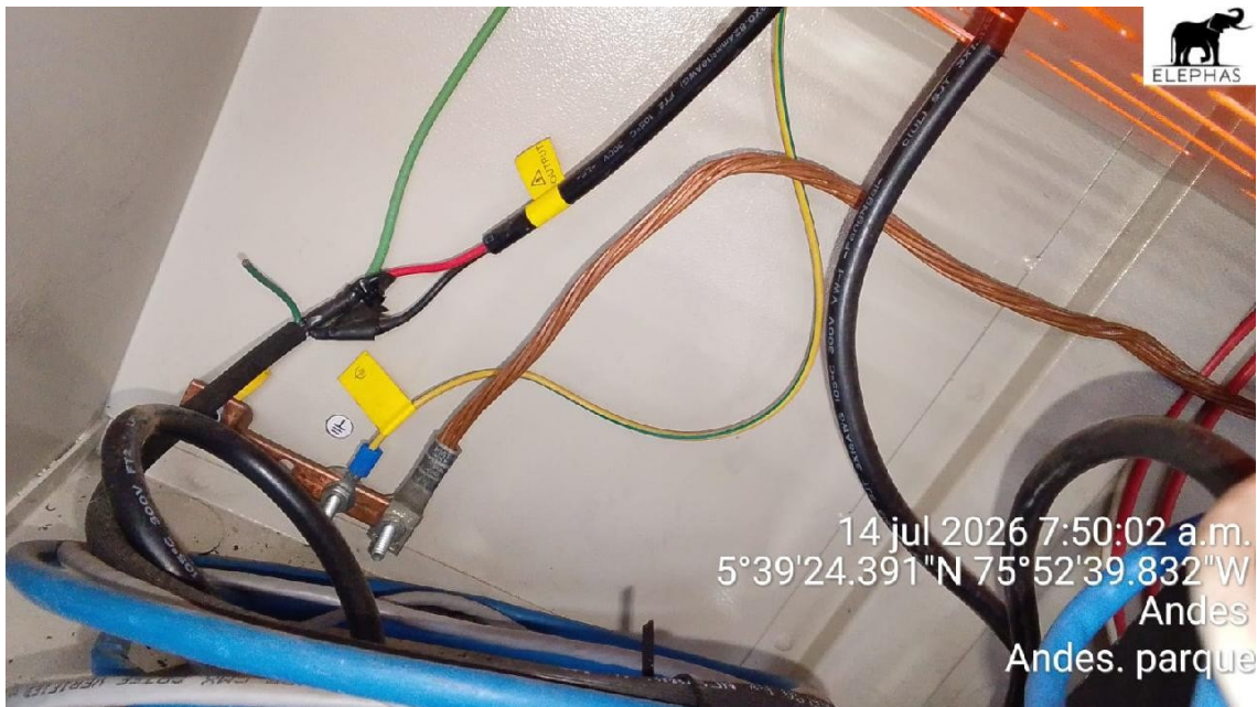
Foto SPT
