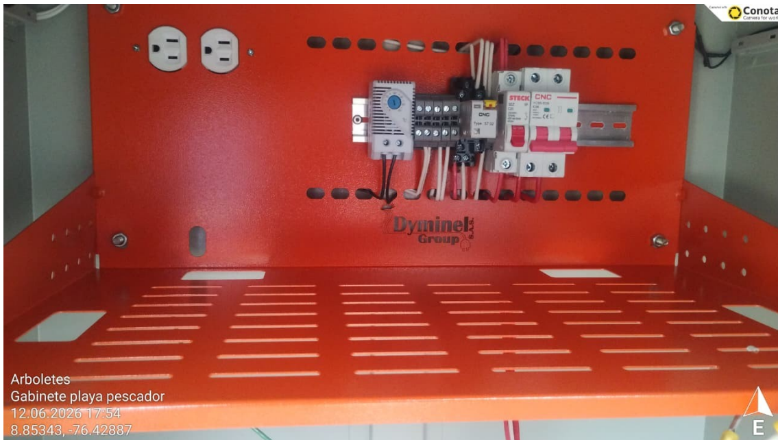
Foto Tablero Breaker
