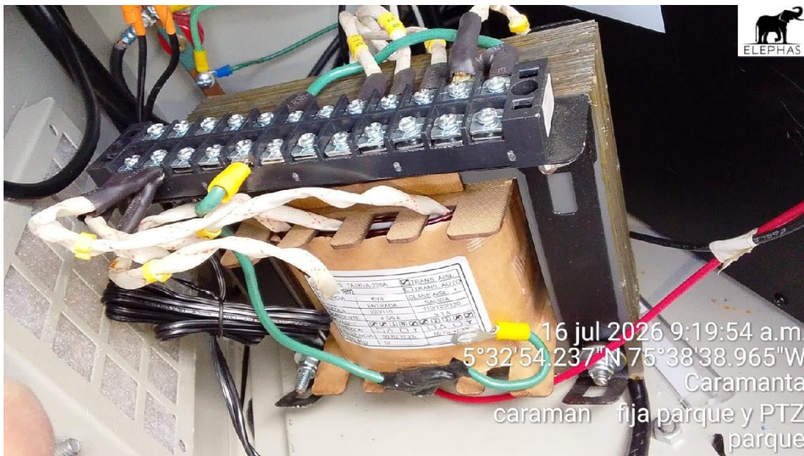
Foto Transformador Reductor
