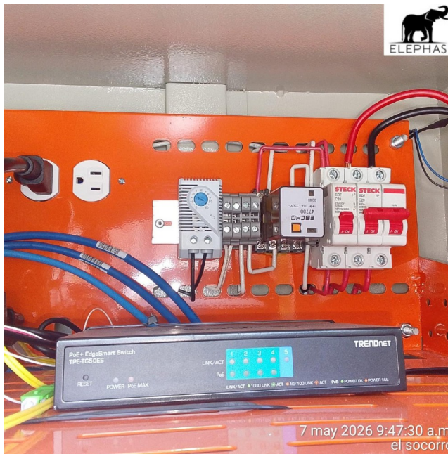
Foto Cables
