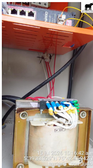
Foto Transformador Reductor
