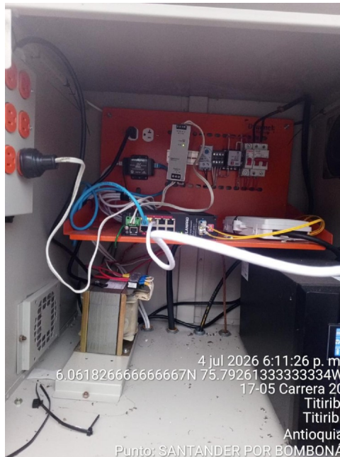
Foto Toma 125 V
