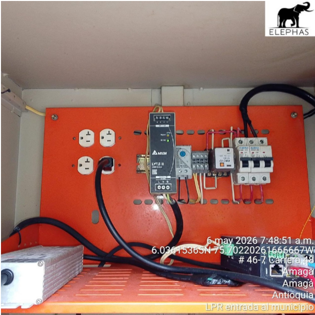
Foto Toma 125 V
