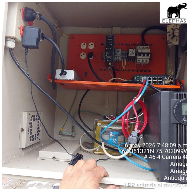
Foto Transformador Reductor
